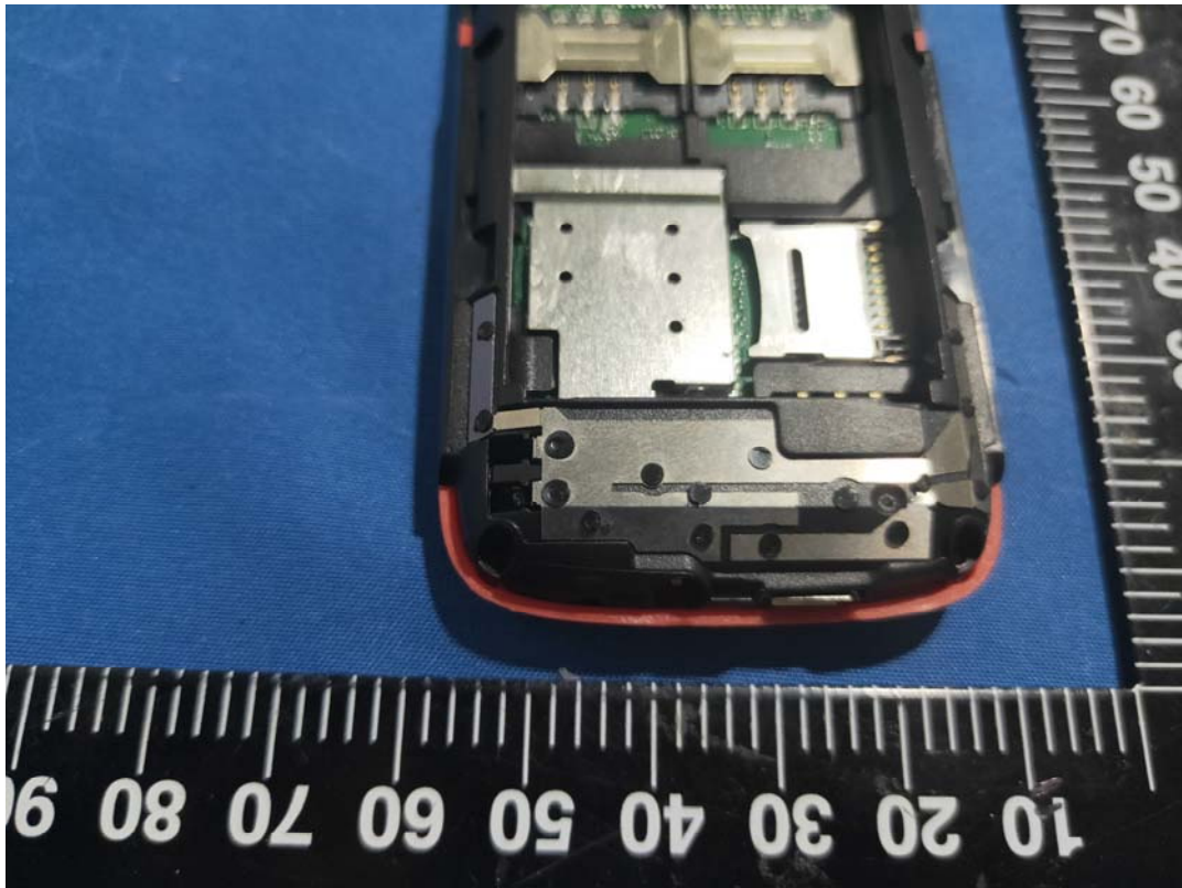
GSM Antenna
