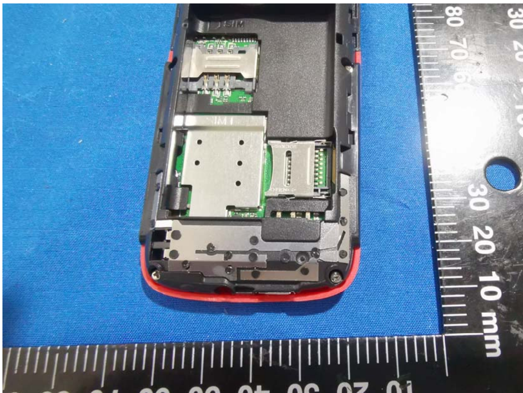
GSM Antenna
