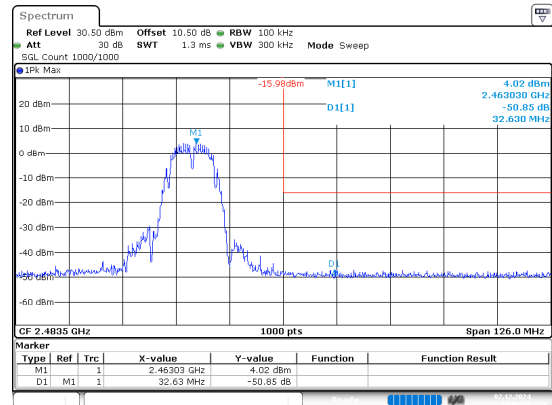
802.11b_2462MHz
