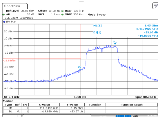
802.11n20_2412MHz
