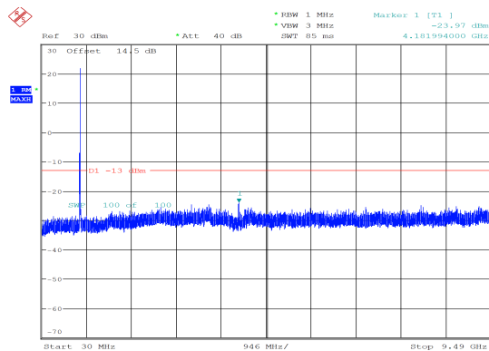
5MHz_Middle_QPSK_25@0 -23.97 dBm
