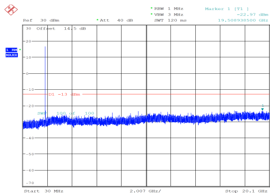
10MHz_Low_QPSK_50@0 -22.97 dBm
