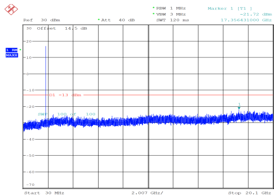
5MHz_Low_QPSK_25@0 -21.72 dBm
