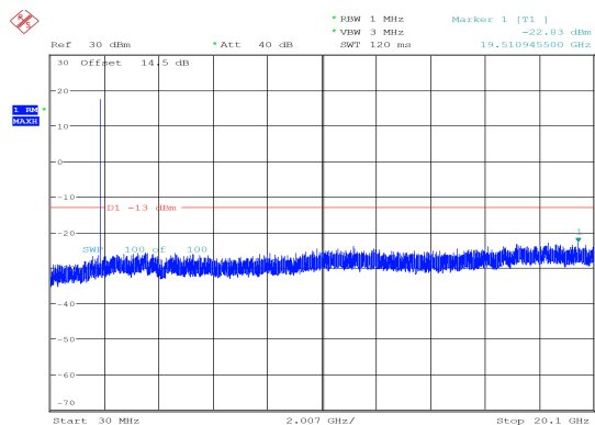
5MHz_Middle_QPSK_25@0 -22.83 dBm
