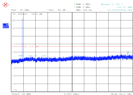
5MHz_Low_QPSK_1@24 -22.37 dBm
