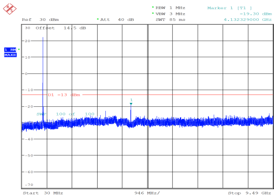
5MHz_Low_QPSK_25@0 -19.30 dBm
