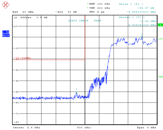
\pi/4 -DQPSK_Hopping_Lower 49.97 dB
