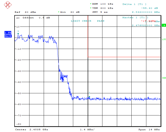
\pi/4 -DQPSK_Hopping_Upper 55.40 dB
