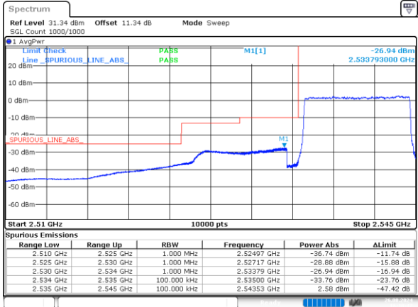
2_10MHz_Low_QPSK_50@0
