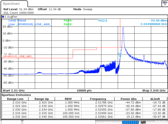
2_10MHz_Low_QPSK_1@0
