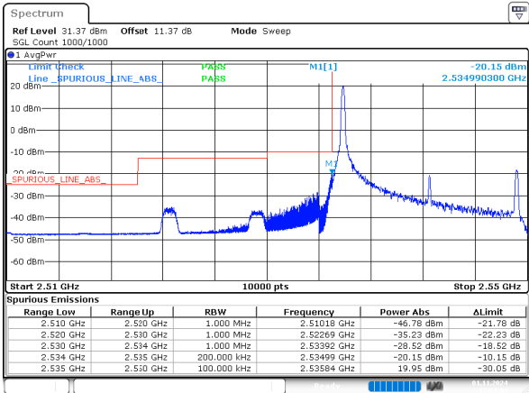
2_15MHz_Low_QPSK_1@0
