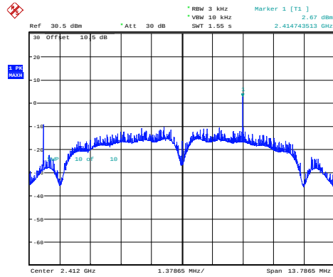
b_2412MHz_Chain 0 2.67dBm/3kHz
