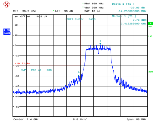
g_2412MHz_Chain 0 30.06dB
