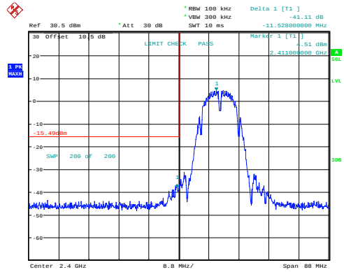
b_2412MHz_Chain 0 41.11dB
