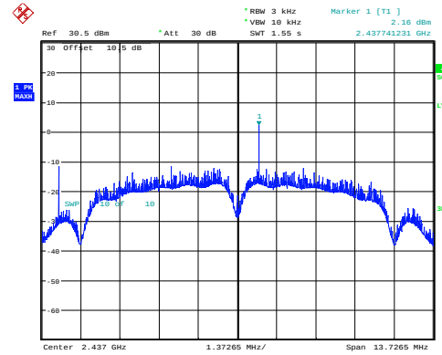
b_2437MHz_Chain 0 2.16dBm/3kHz
