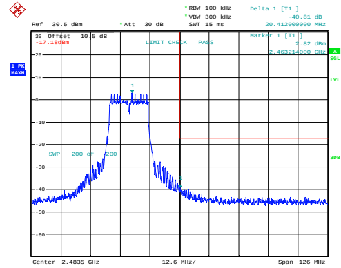
g_2462MHz_Chain 0 40.81dB
