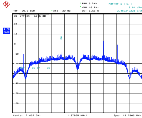
b_2462MHz_Chain 0 3.84dBm/3kHz
