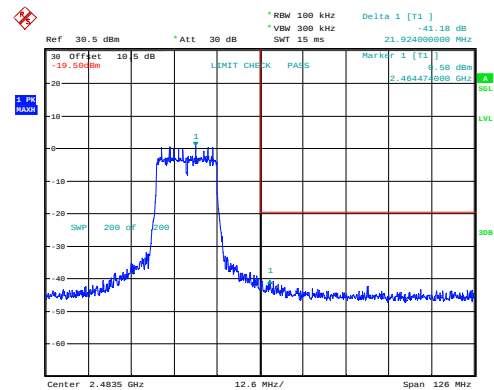
n20_2462MHz_Chain 0 41.18dB
