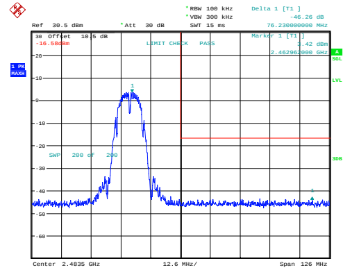
b_2462MHz_Chain 0 46.26dB
