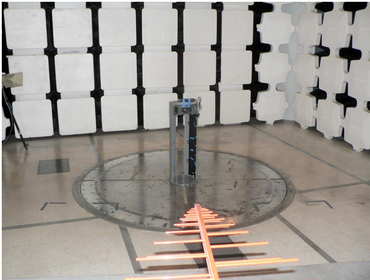
LYFT18 Digital Emissions 30-1000MHz
