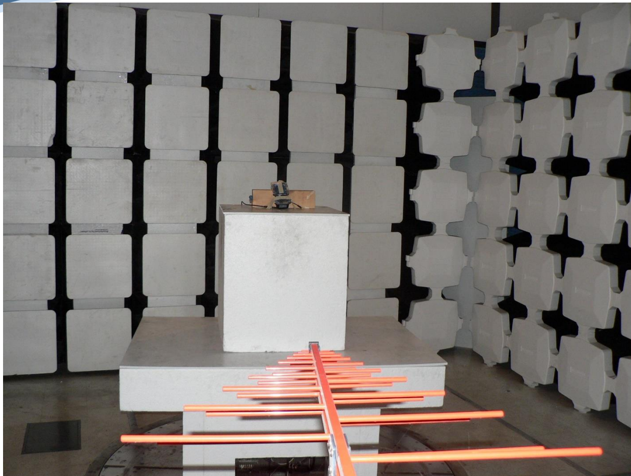
LYFT08 TX Spurious 30-1000MHz
