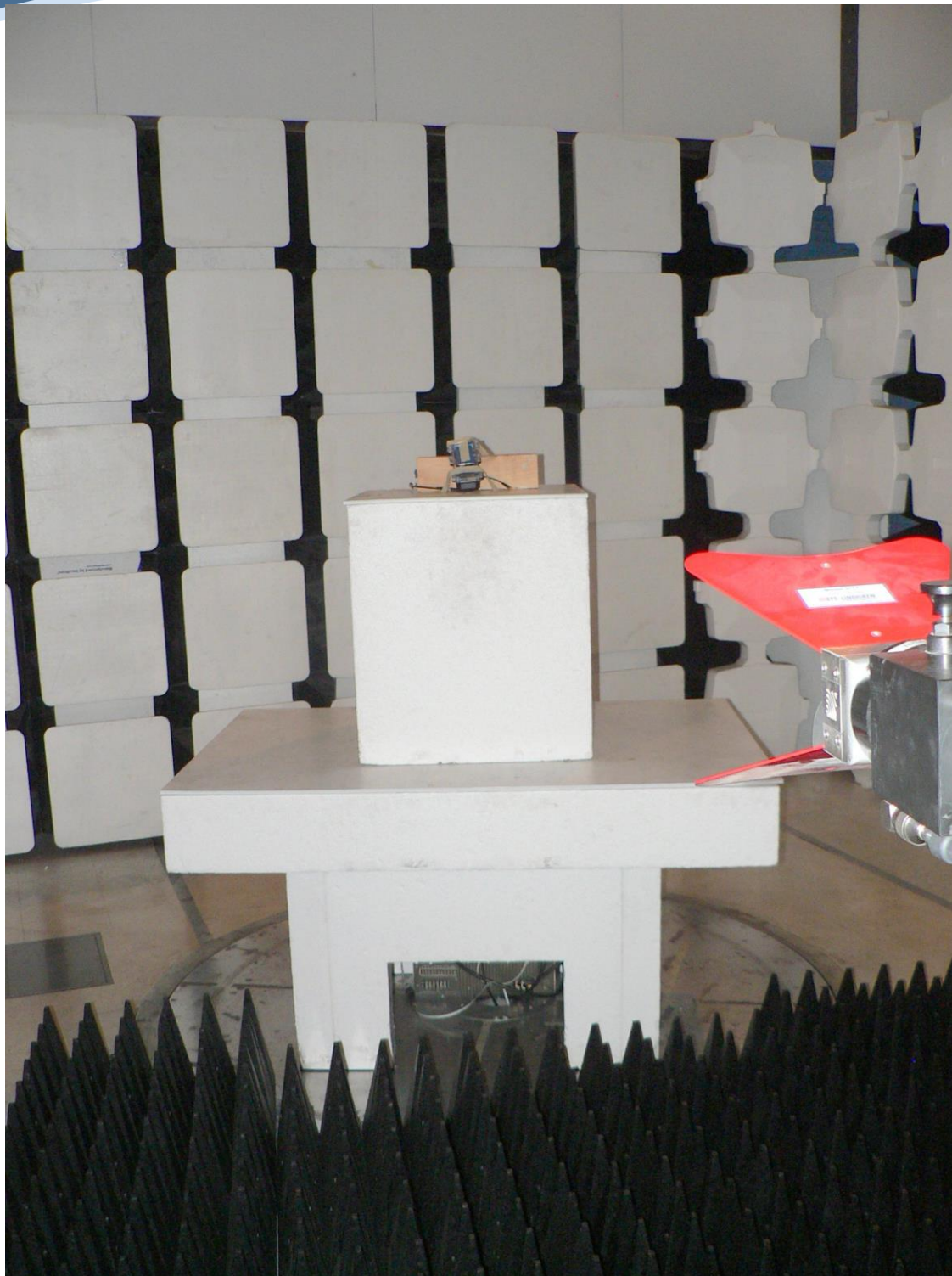
LYFT08 TX Spurious 1-18GHz
