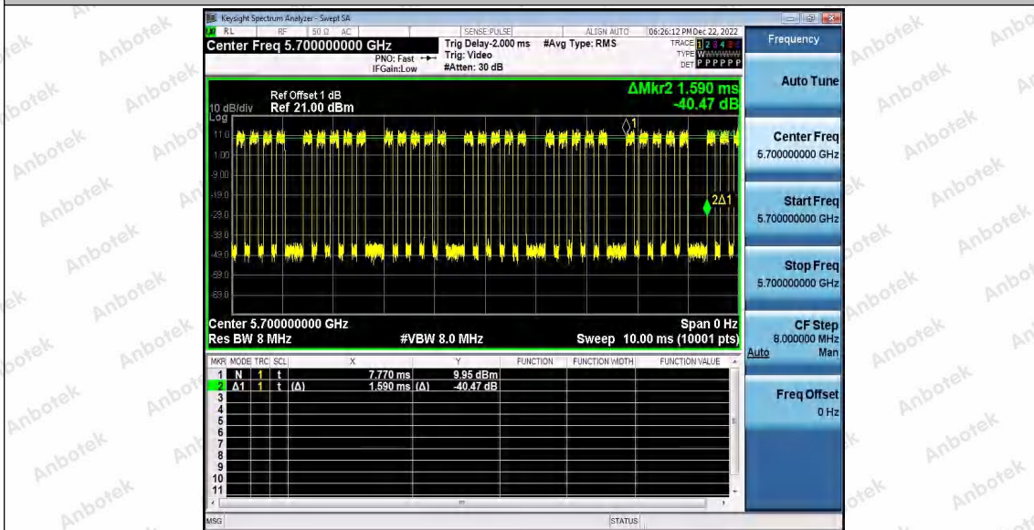
11N20SISO_Ant2_5700
