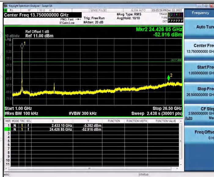
11N40_Ant1_2437_0~Reference
