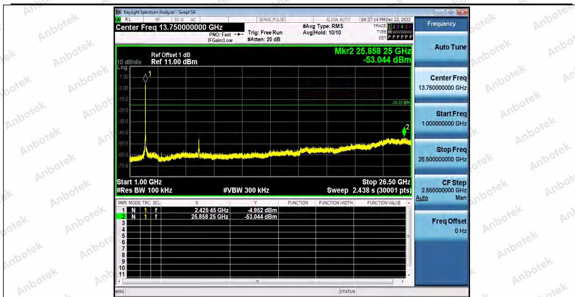
11N40_Ant2_2422_0~Reference
