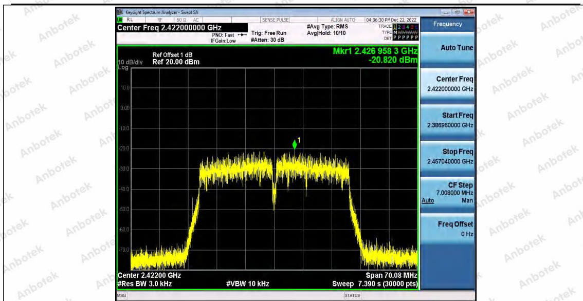
11N40_Ant2_2422
