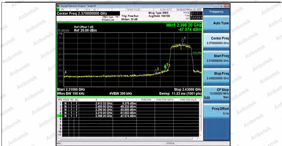
11N20_Ant2_Low_2412
