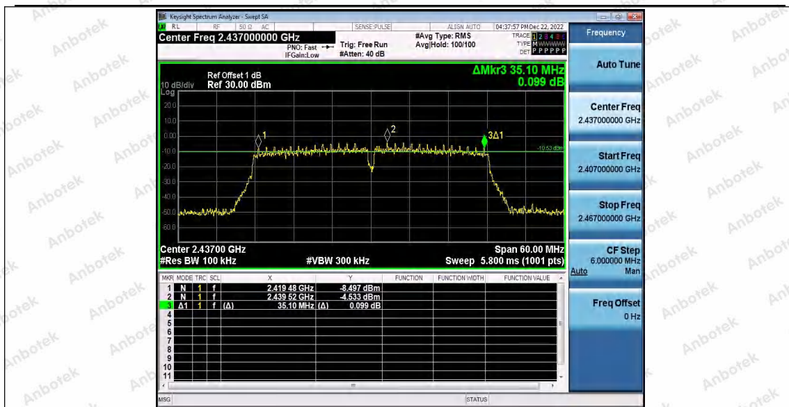
11N40_Ant2_2437
