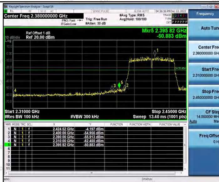
11N40_Ant2_Low_2422
