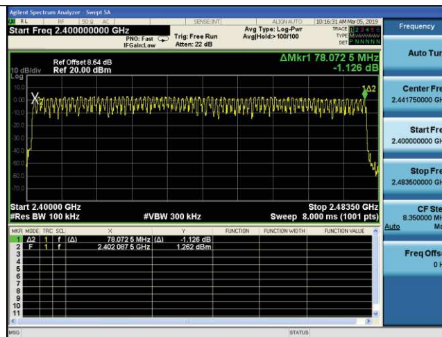
\pi/4 DQPSK
