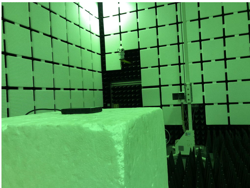
Fig. 2 (Above 1GHz)
