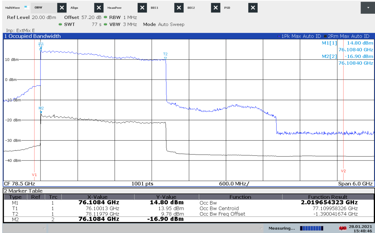
Plot 68: OBW, +40 °C / V_{nom} , Mode 5
