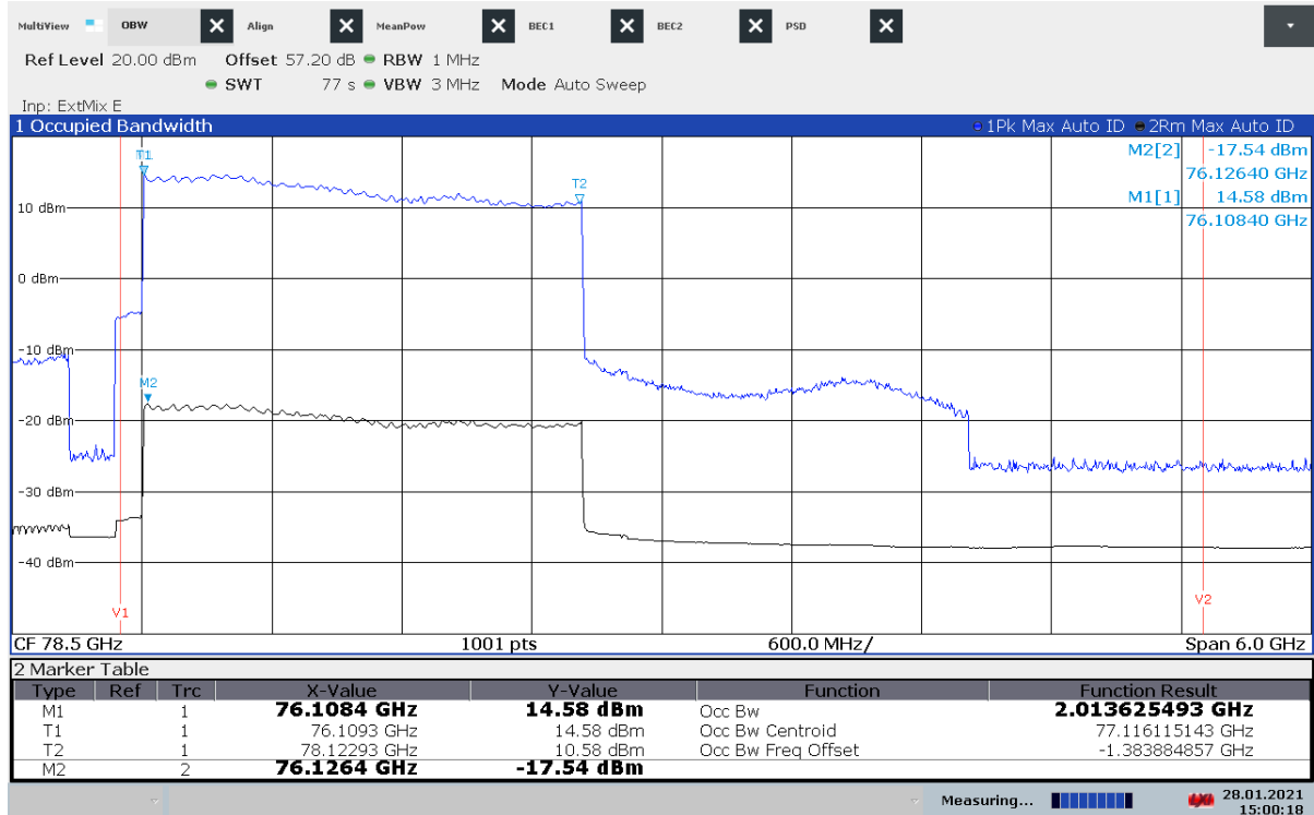
Plot 59: OBW, +10 °C / V nom , Mode 5
