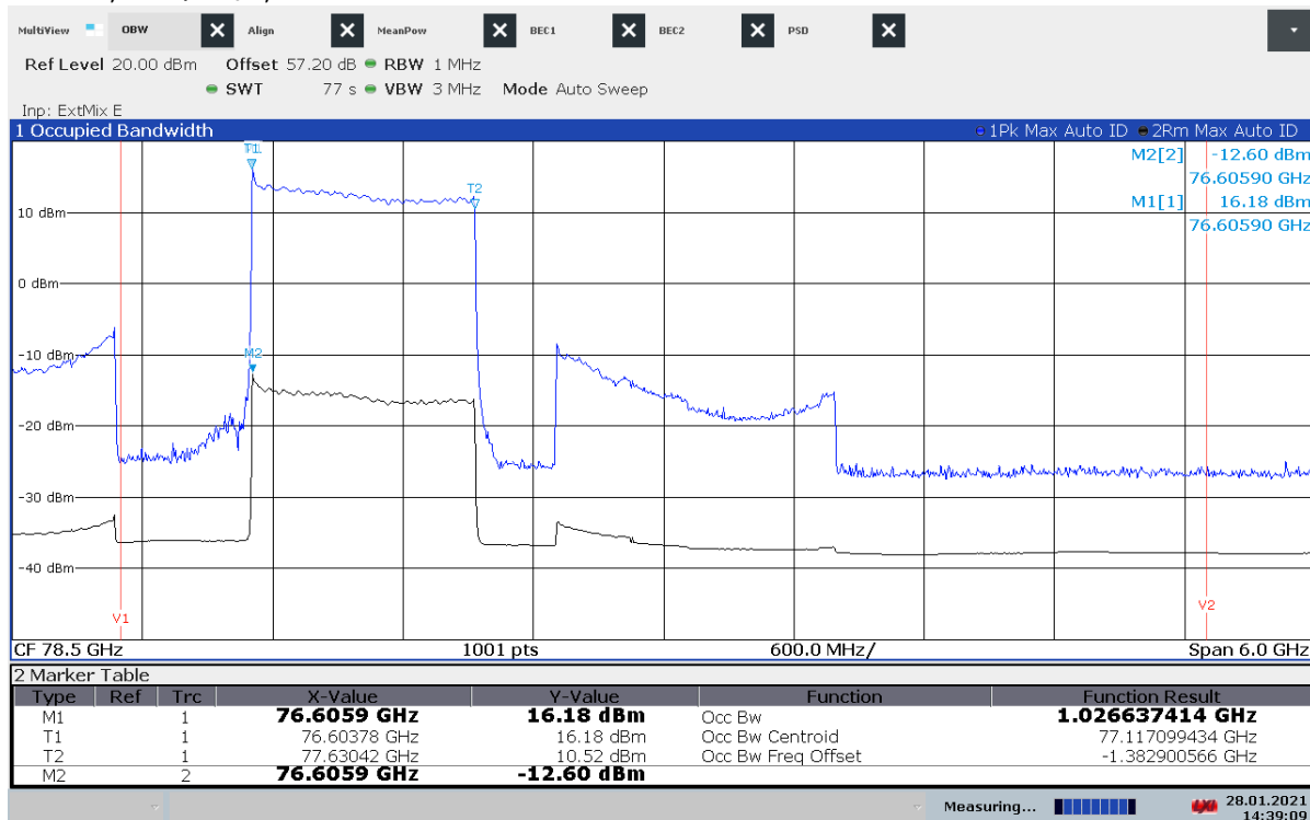
Plot 55: OBW, 0 °C / V nom , Mode 3
