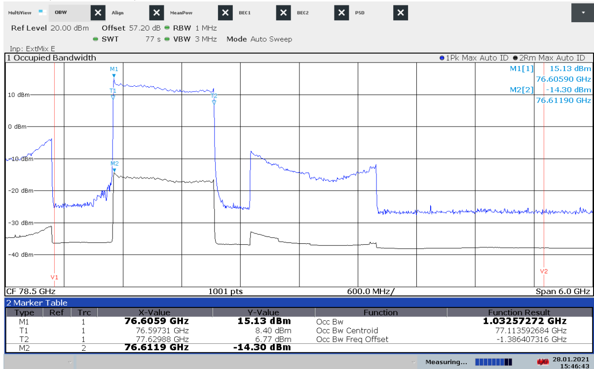
Plot 67: OBW, +40 °C / V_{nom} , Mode 3
