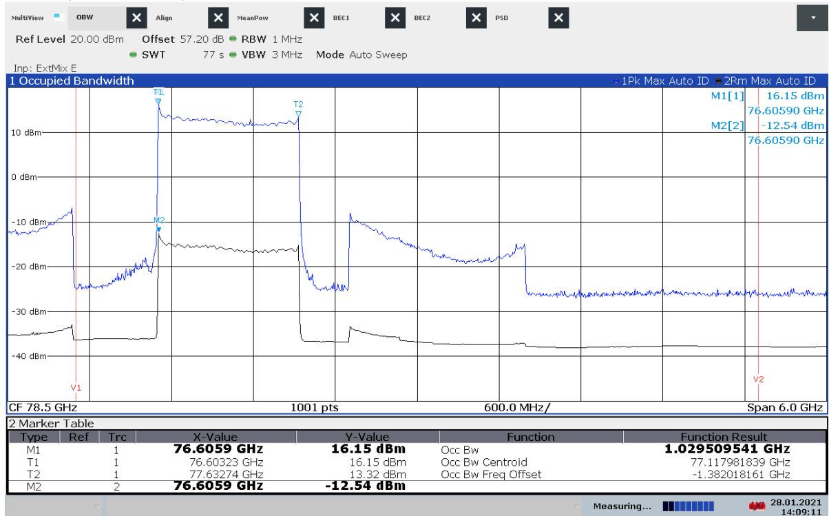
Plot 49: OBW, -20 °C / V nom , Mode 3
