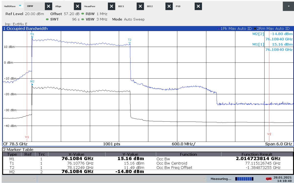
Plot 54: OBW, -10 °C / V nom , Mode 6
