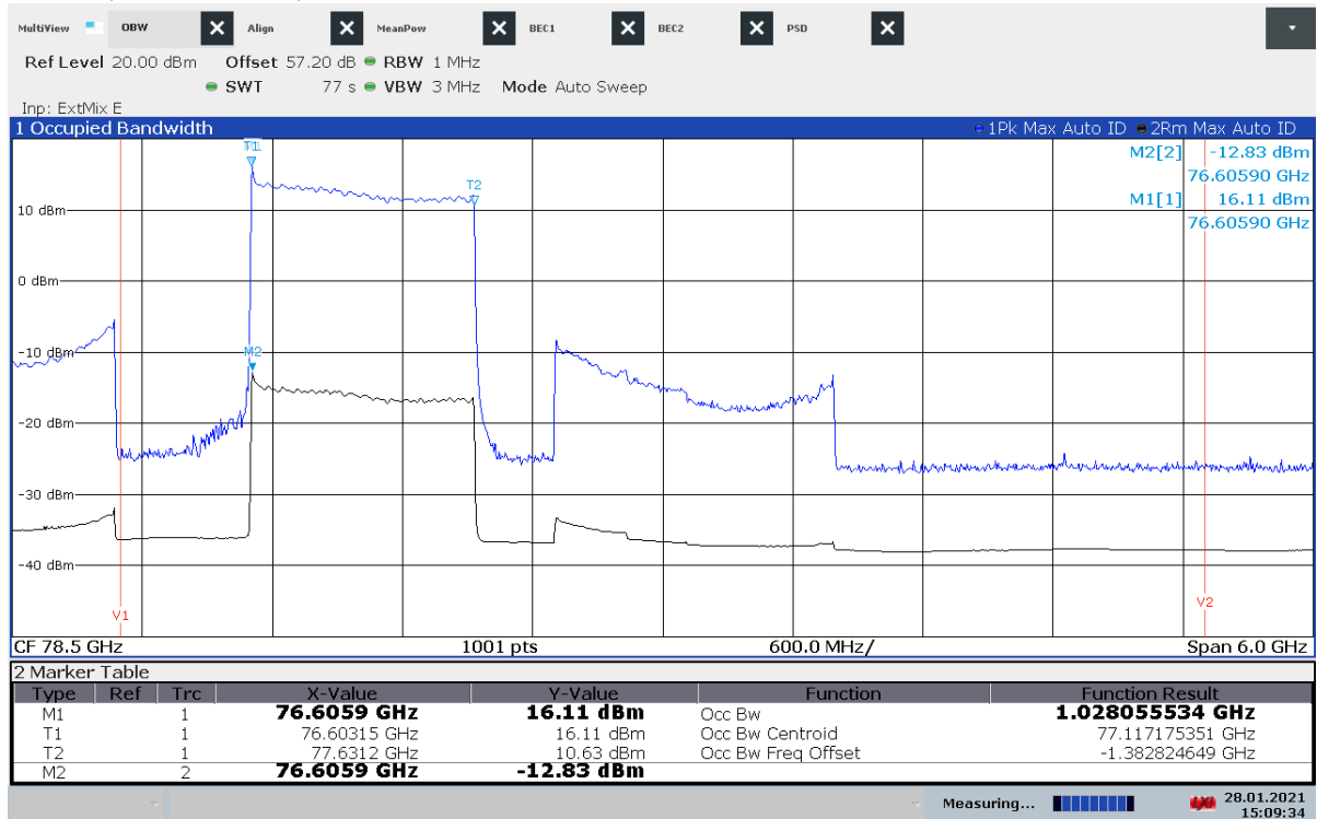
Plot 58: OBW, +10 °C / V nom , Mode 3
