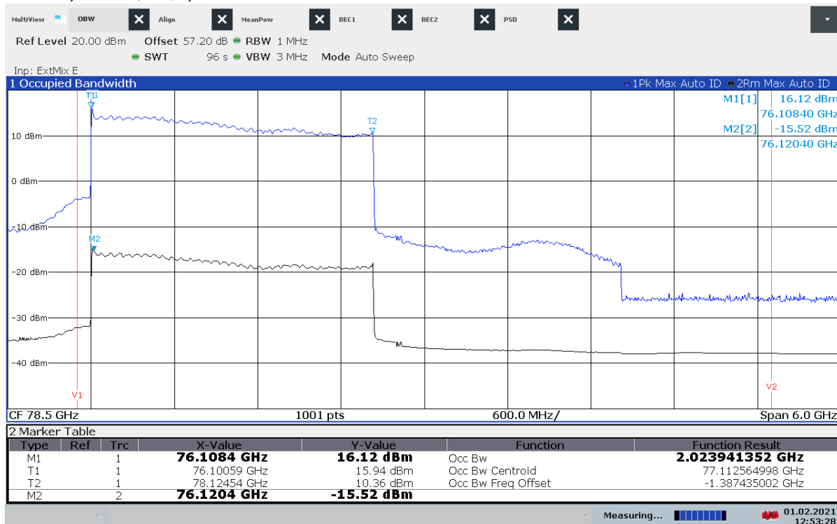
Plot 63: OBW, +20 °C / V nom , Mode 6
