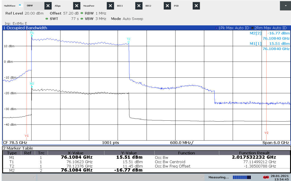
Plot 50: OBW, -20 °C / V nom , Mode 5
