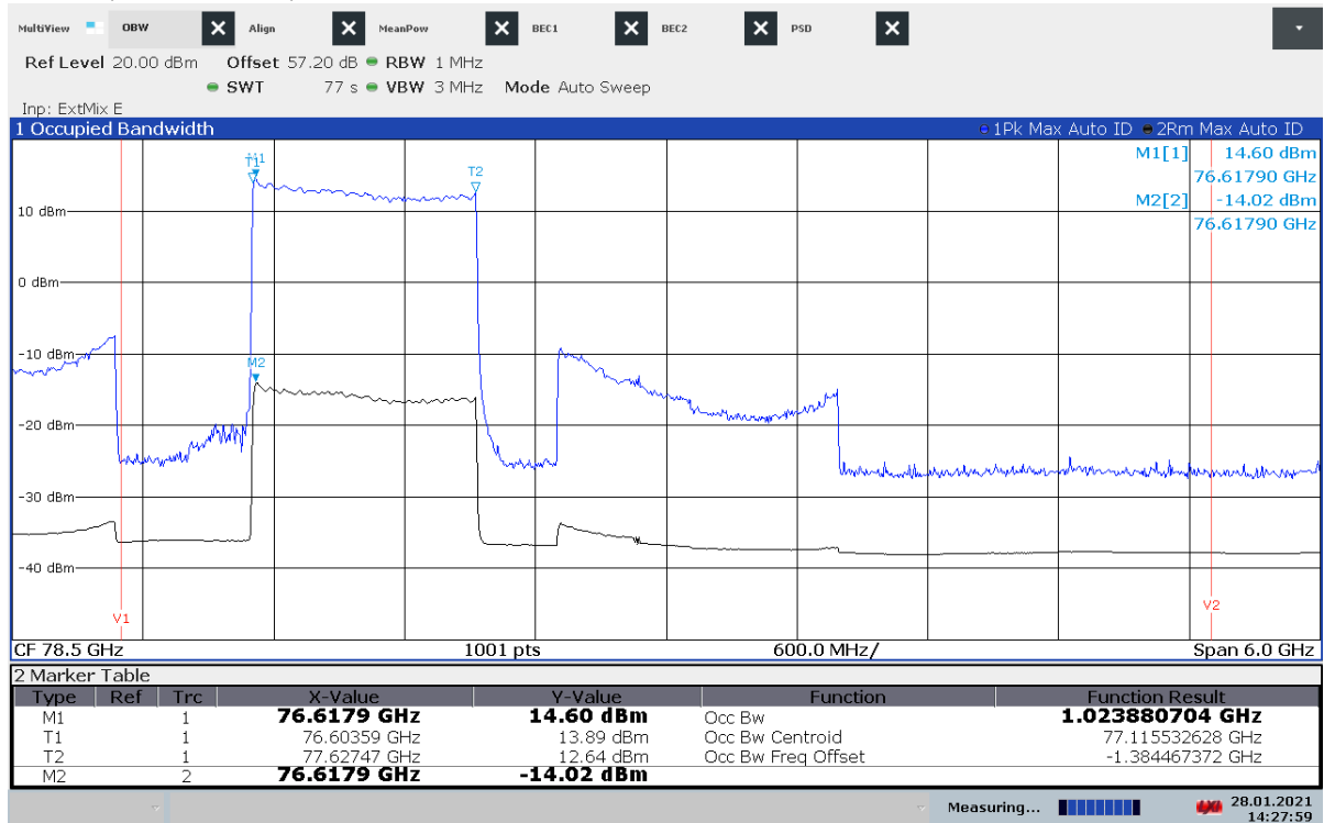
Plot 52: OBW, -10 °C / V nom , Mode 3
