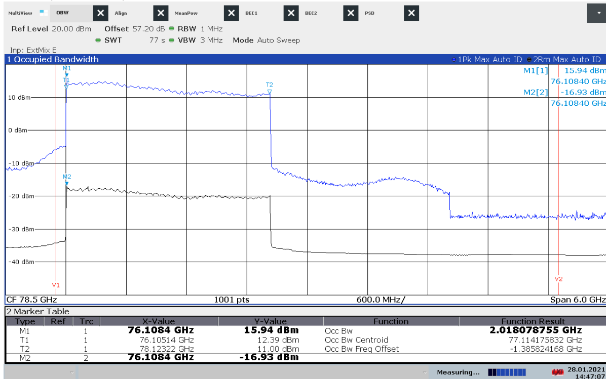
Plot 56: OBW, 0 °C / V nom , Mode 5
