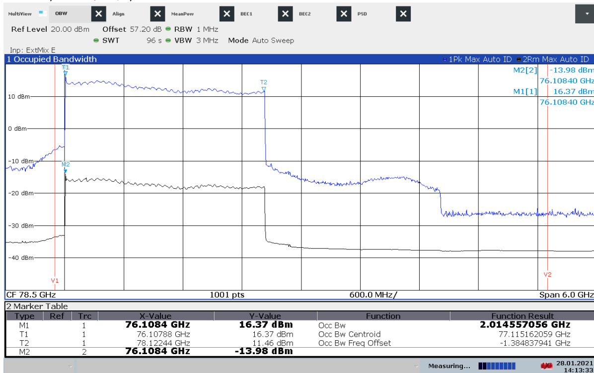
Plot 51: OBW, -20 °C / V nom , Mode 6
