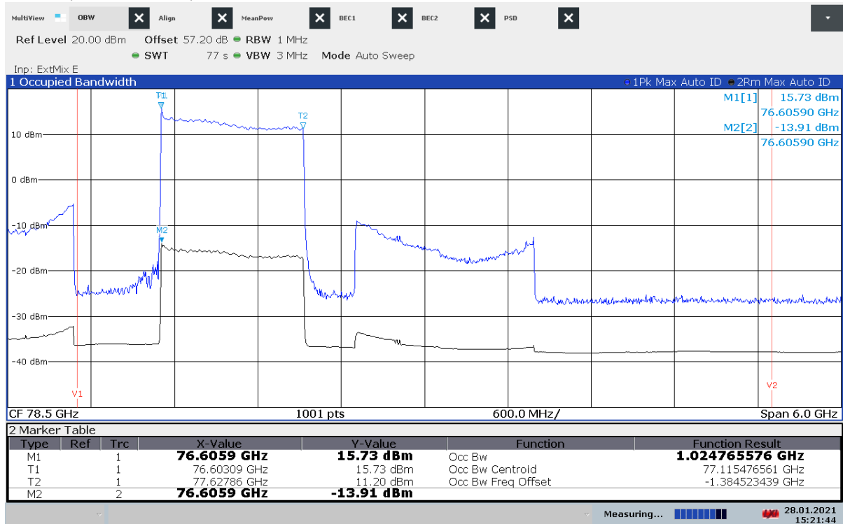
Plot 64: OBW, +30 °C / V_{nom} , Mode 3
