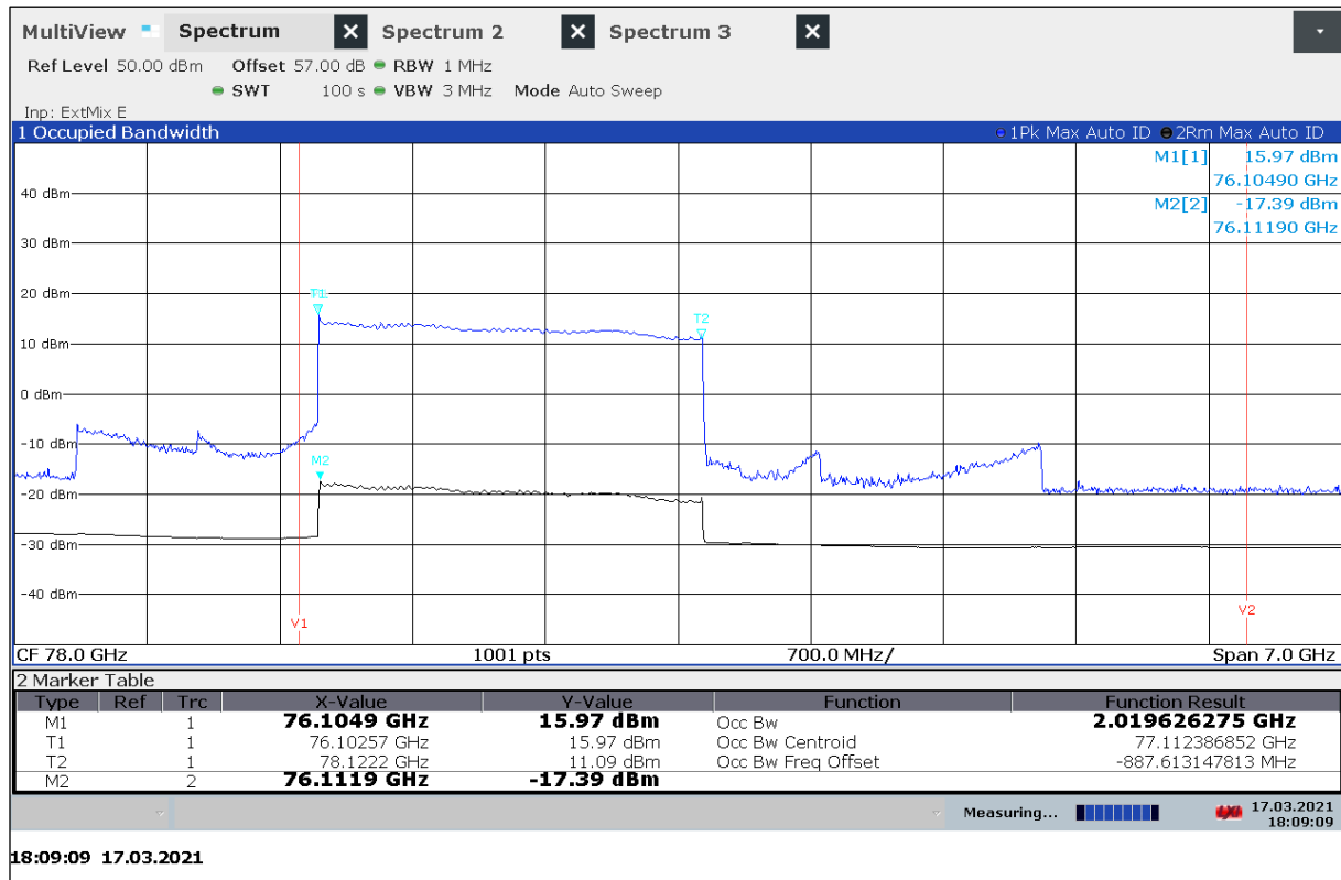
Plot 29: OBW, 40 °C / V nom
