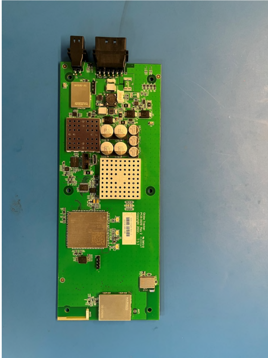
PCB Top
