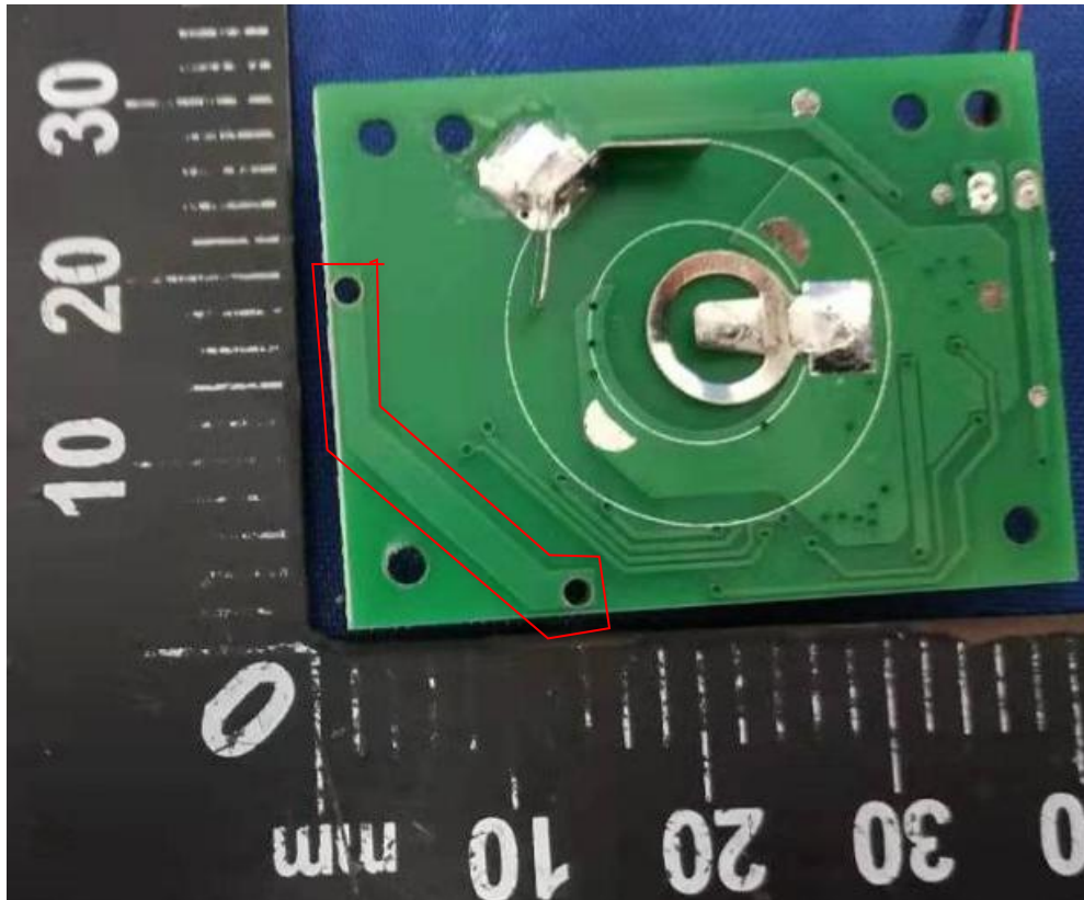
Antenna
