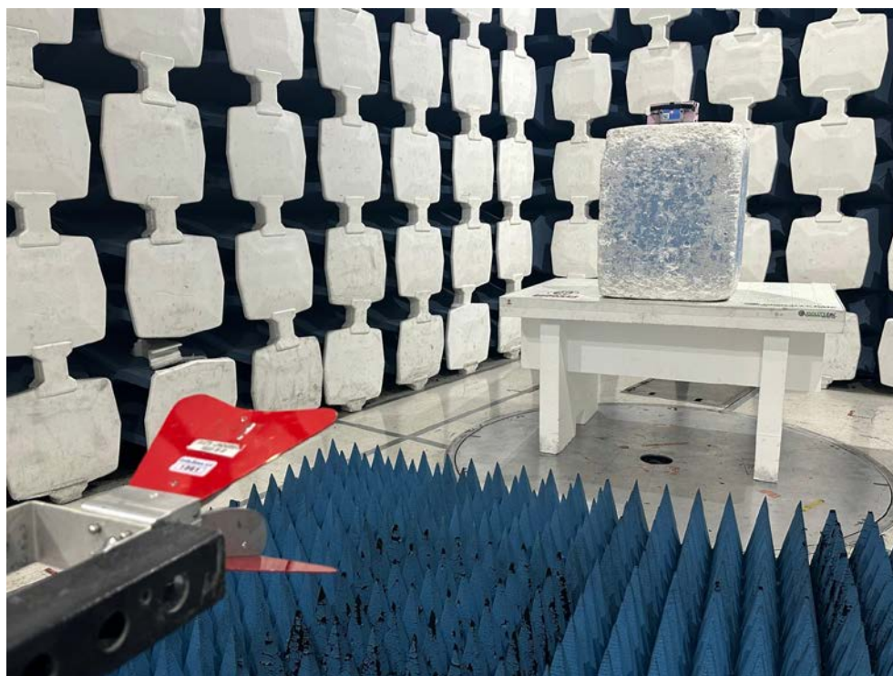
1-18GHz Front
