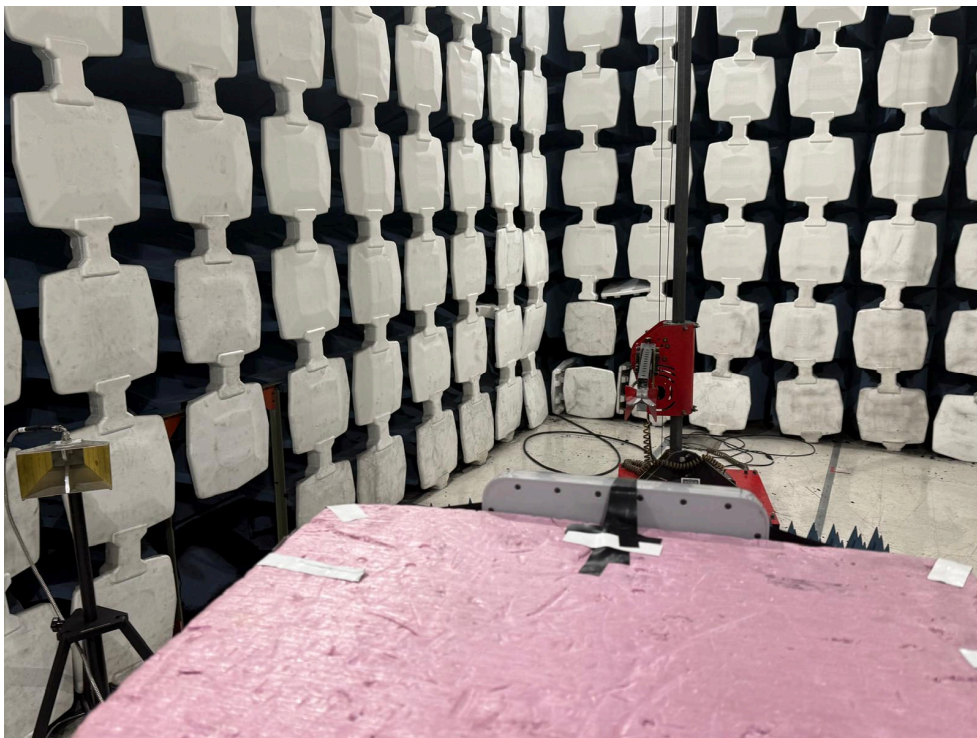
1-18GHz Rear
