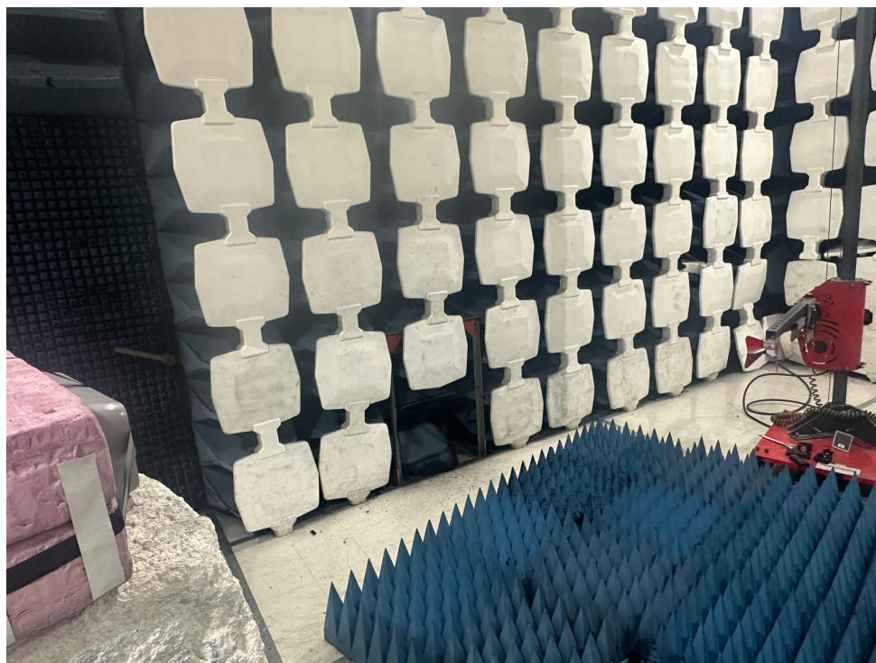
1-18GHz Rear
