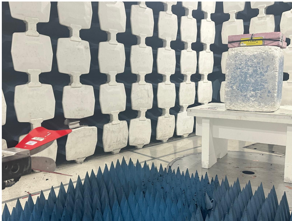
1-18GHz Front
