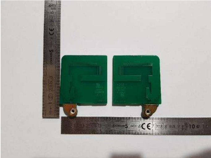
AVW0158 – 5G Antennas
