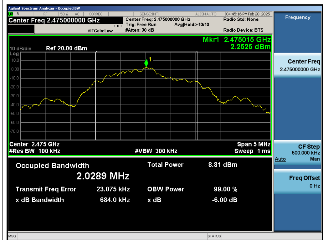
Test_Graph_GFSK_ANT1_2475_DTSBW
