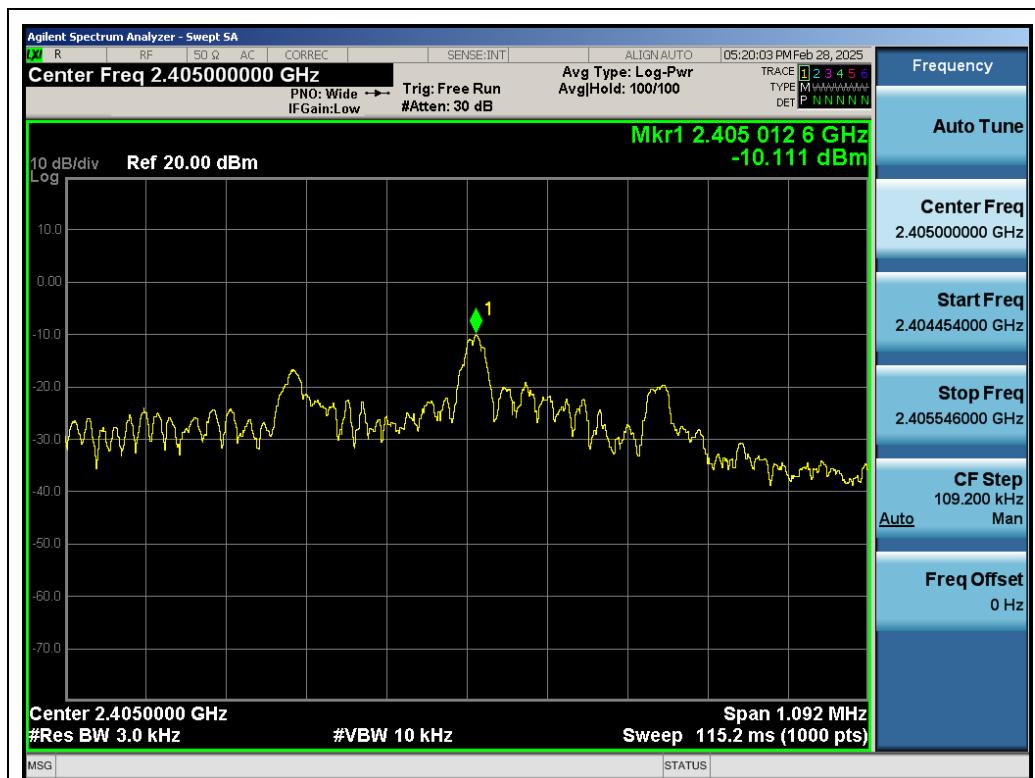
Test_Graph_GFSK_ANT1_2405_PSD
