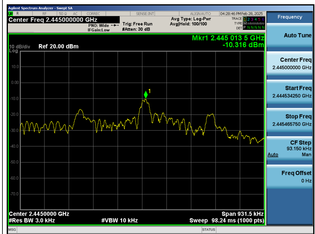
Test_Graph_GFSK_ANT1_2445_PSD
