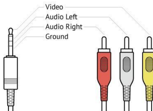
Mini Jack – A/V Cable
