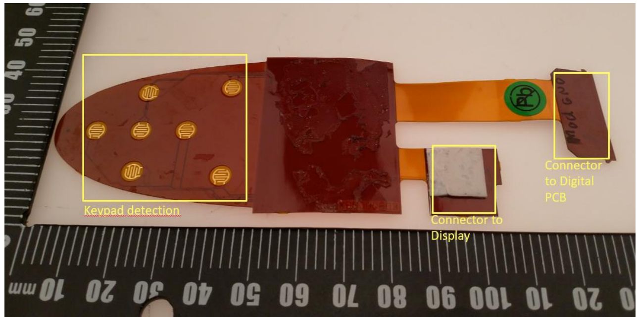
ZD0921. Display / Keyboard PCB. Top side
