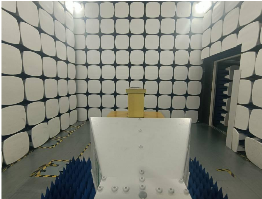
1GHz - 18GHz
