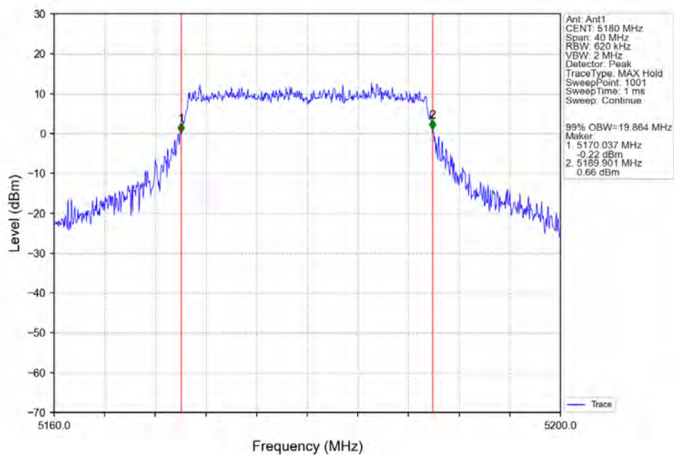
802.11ax(HE20) LCH 5180MHz SU / Ant1 NTN
