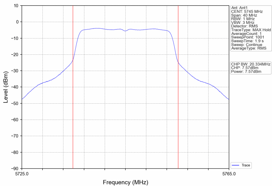
802.11n(HT20)_LCH_5745MHz_Ant1_NTV
