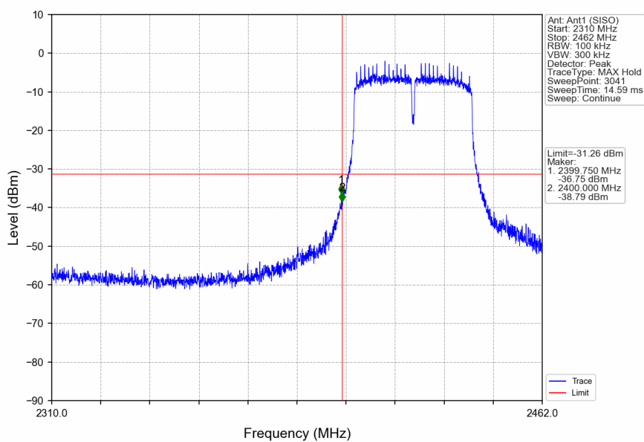
802.11n(HT40) LCH 2422MHz Ant1 (SISO) NTNV
