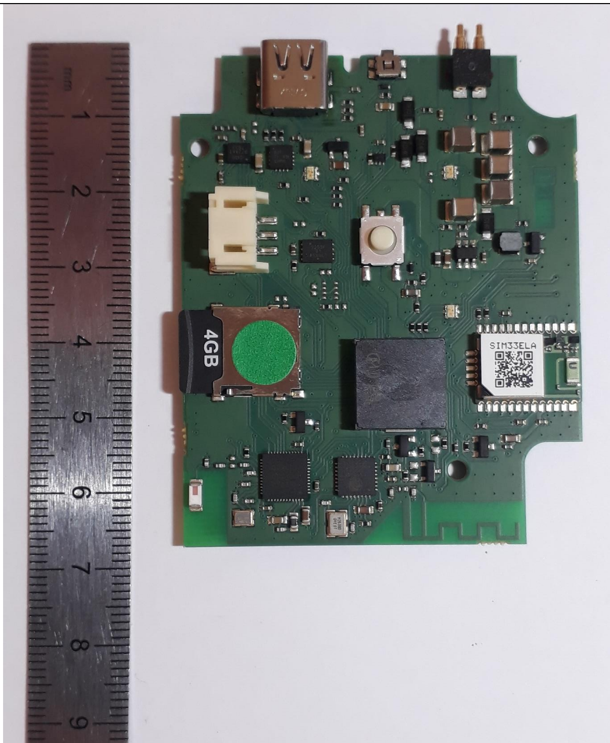
PCBA Bottom
