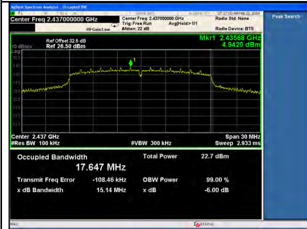
11n-20MHz-6dB BW-Mid-MCS0
