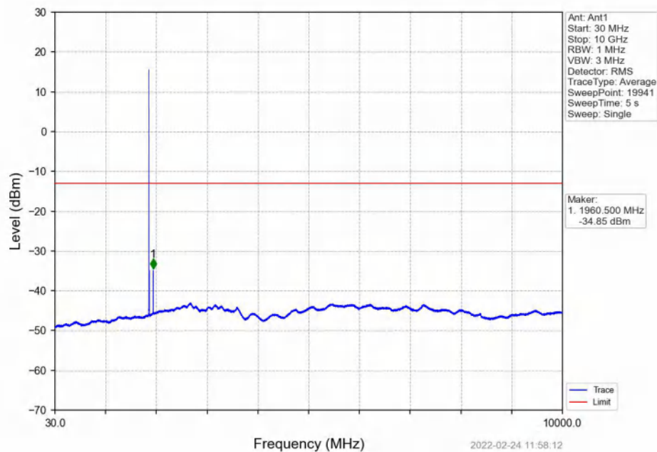
Band2_5MHz_QPSK_MCH_1880MHz_RB_1_0_NTNV
