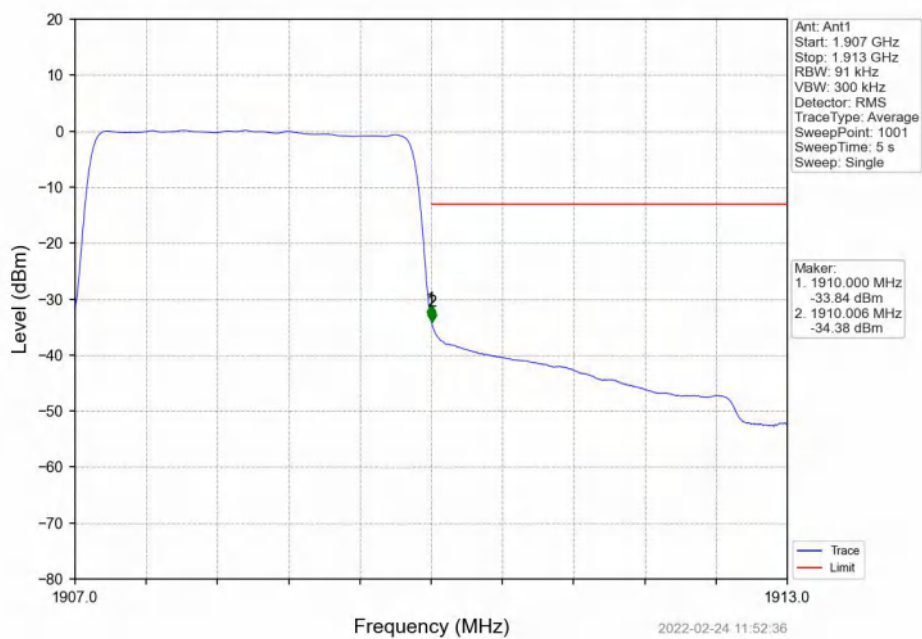
Band2_3MHz_QPSK_HCH_1908.5MHz_RB_15_0_NTNV
