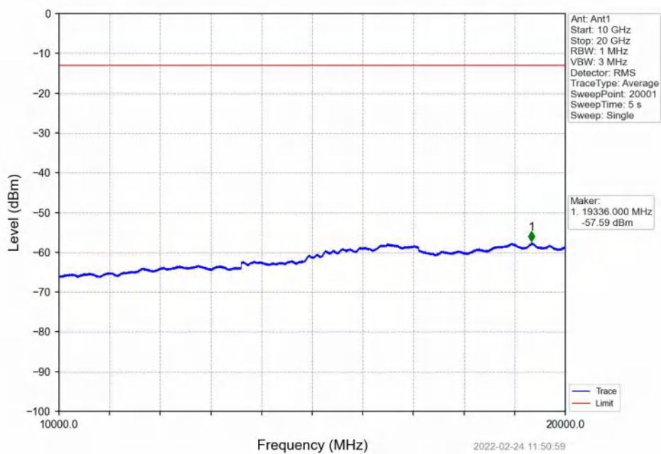
Band2_3MHz_16QAM_MCH_1880MHz_RB_1_0_NTNV
