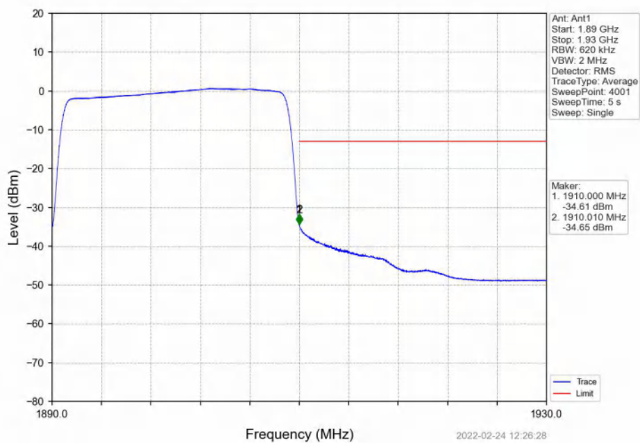
Band2_20MHz_QPSK_HCH_1900MHz_RB_100_0_NTNV
