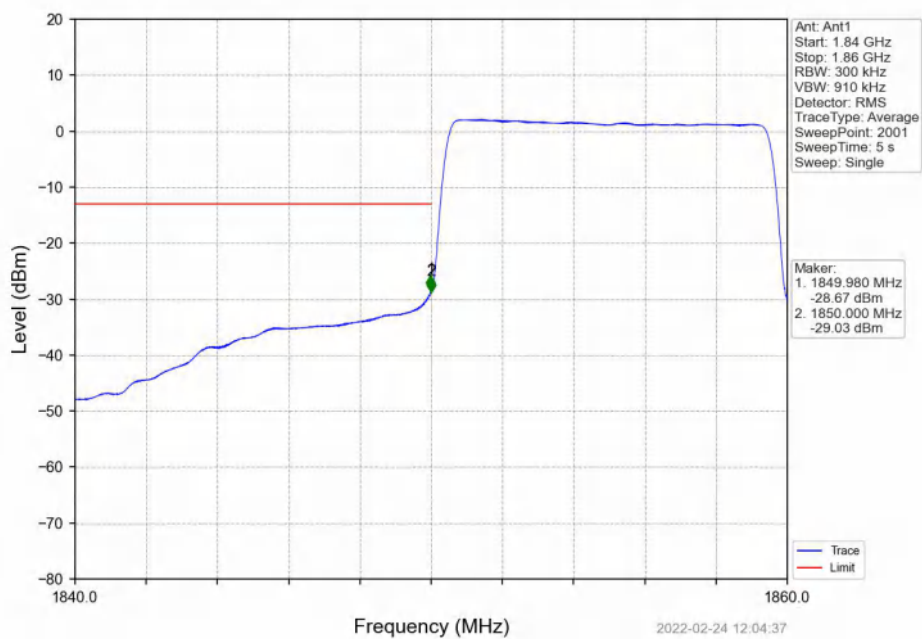
Band2_10MHz_QPSK_LCH_1855MHz_RB_50_0_NTNV
