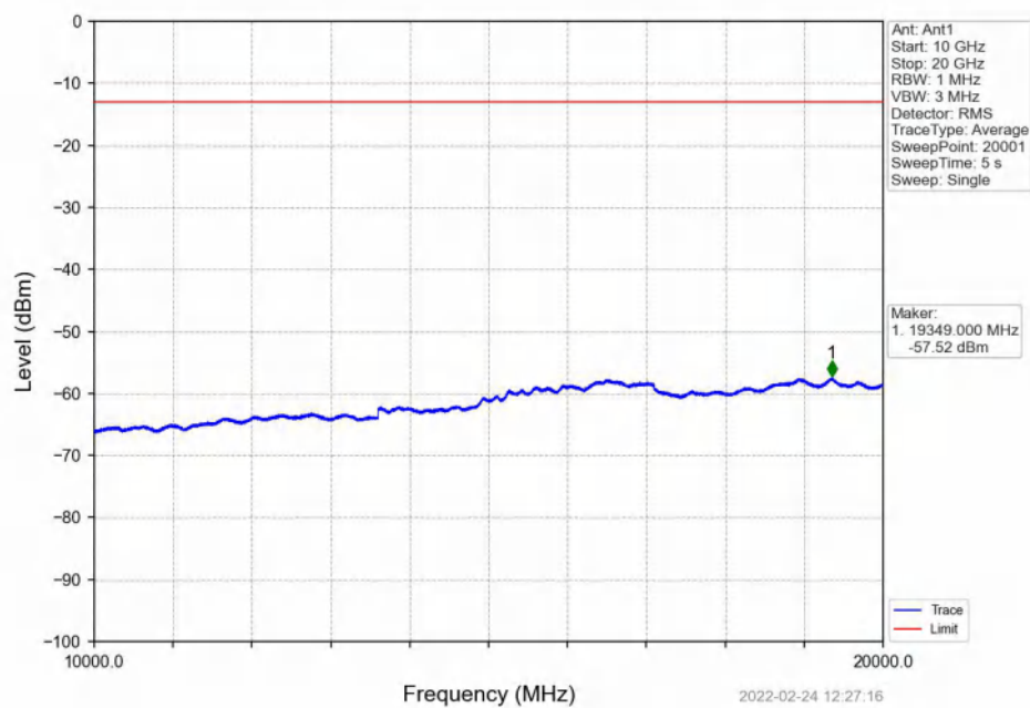
Band2_20MHz_16QAM_HCH_1900MHz_RB_1_0_NTNV
