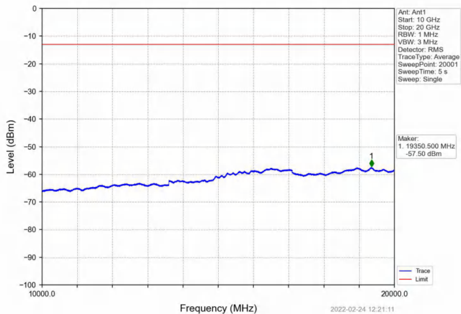
Band2_20MHz_QPSK_LCH_1860MHz_RB_100_0_NTNV
