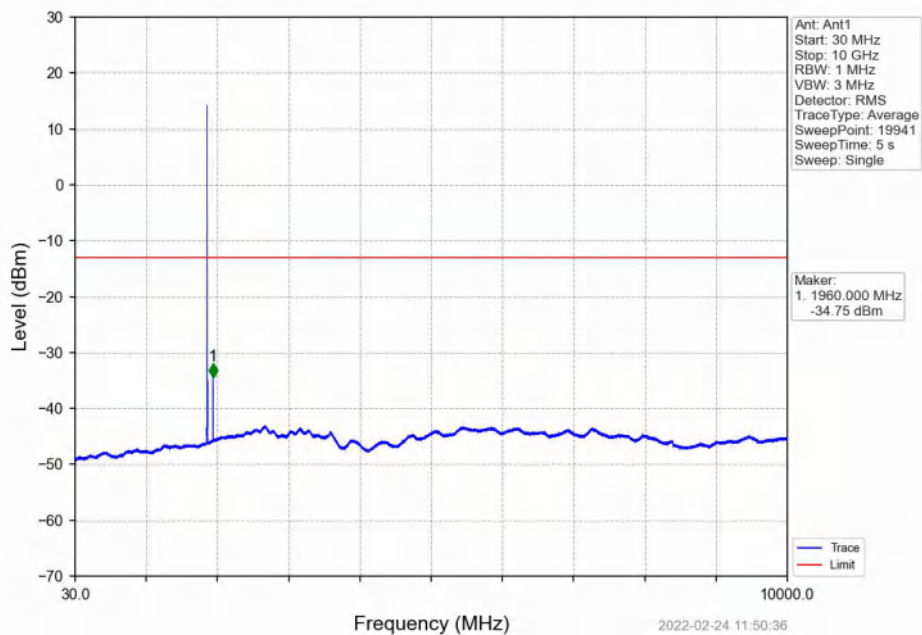
Band2_3MHz_16QAM_MCH_1880MHz_RB_1_0_NTNV
