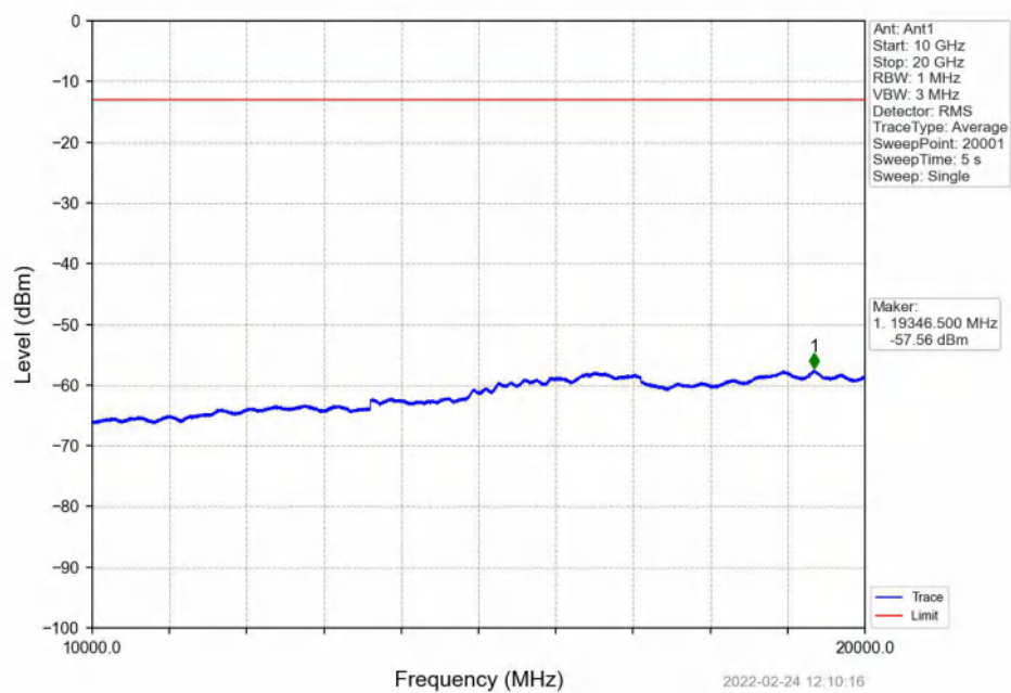
Band2_10MHz_16QAM_HCH_1905MHz_RB_1_0_NTNV
