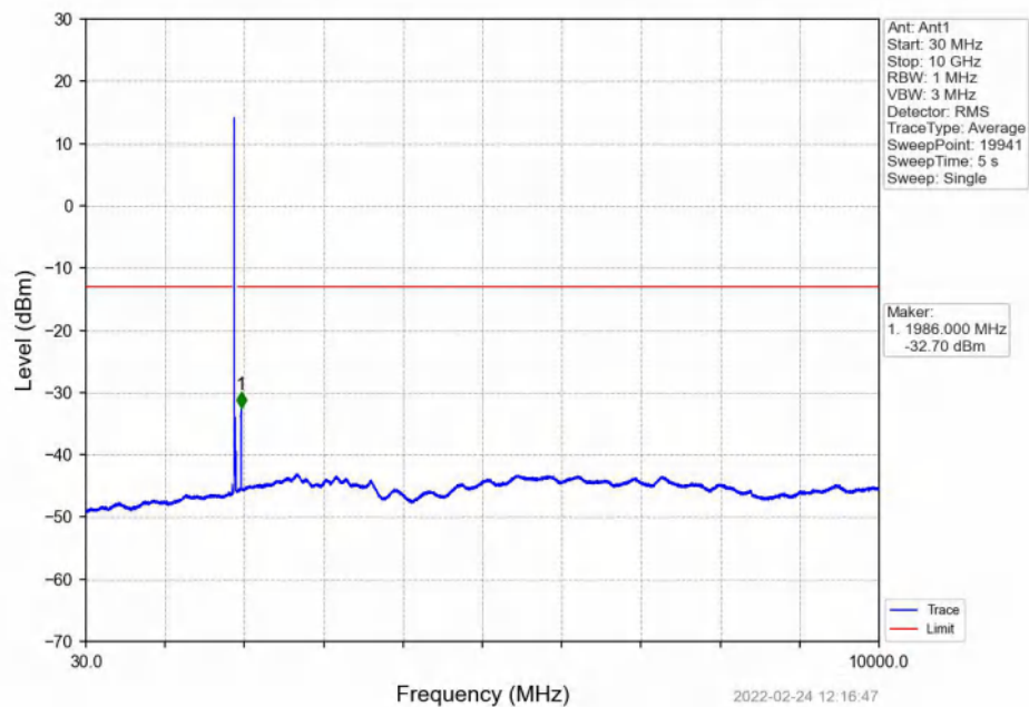
Band2_15MHz_QPSK_HCH_1902.5MHz_RB_1_0_NTNV
