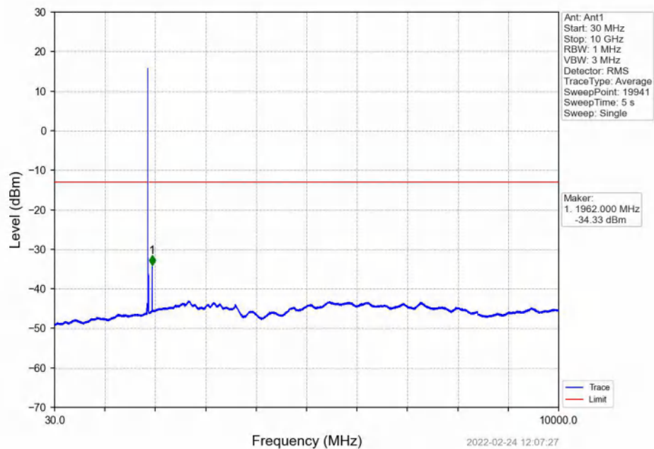
Band2_10MHz_16QAM_MCH_1880MHz_RB_1_0_NTNV
