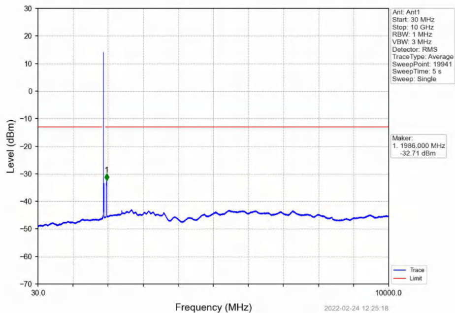
Band2_20MHz_QPSK_HCH_1900MHz_RB_1_0_NTNV
