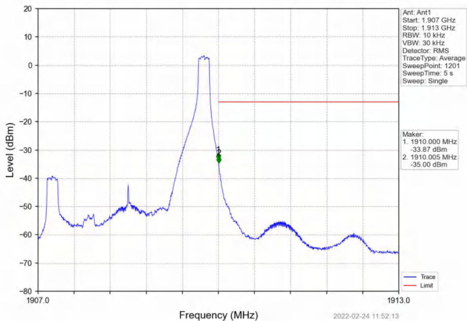
Band2_3MHz_QPSK_HCH_1908.5MHz_RB_15_0_NTNV
