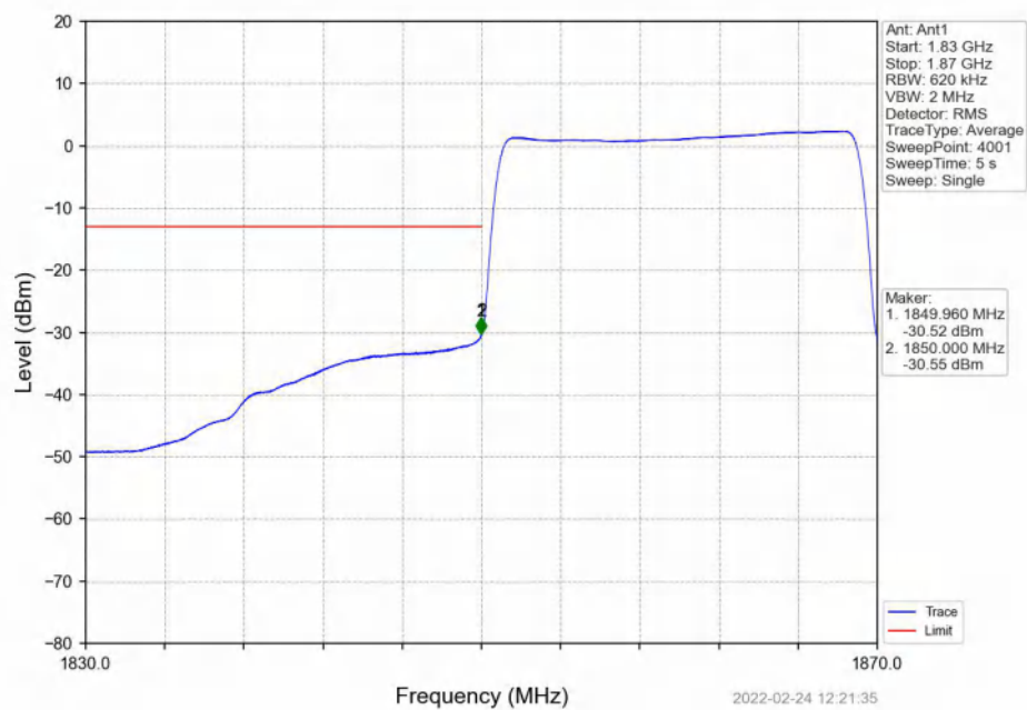
Band2_20MHz_QPSK_LCH_1860MHz_RB_100_0_NTNV
