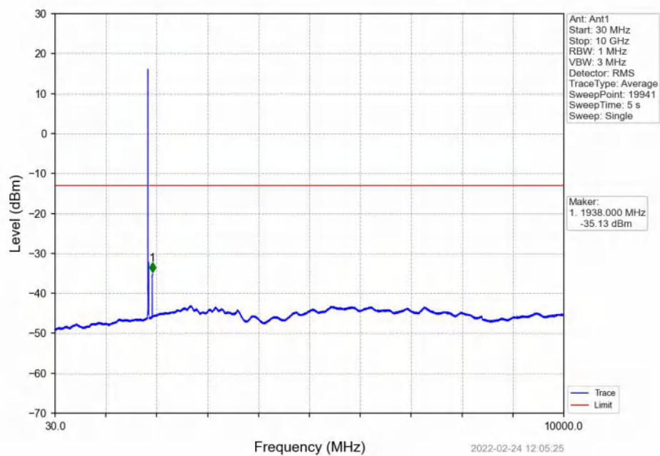
Band2_10MHz_16QAM_LCH_1855MHz_RB_1_0_NTNV
