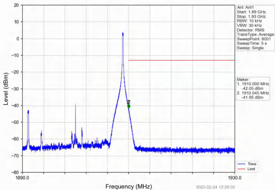
Band2_20MHz_QPSK_HCH_1900MHz_RB_100_0_NTNV
