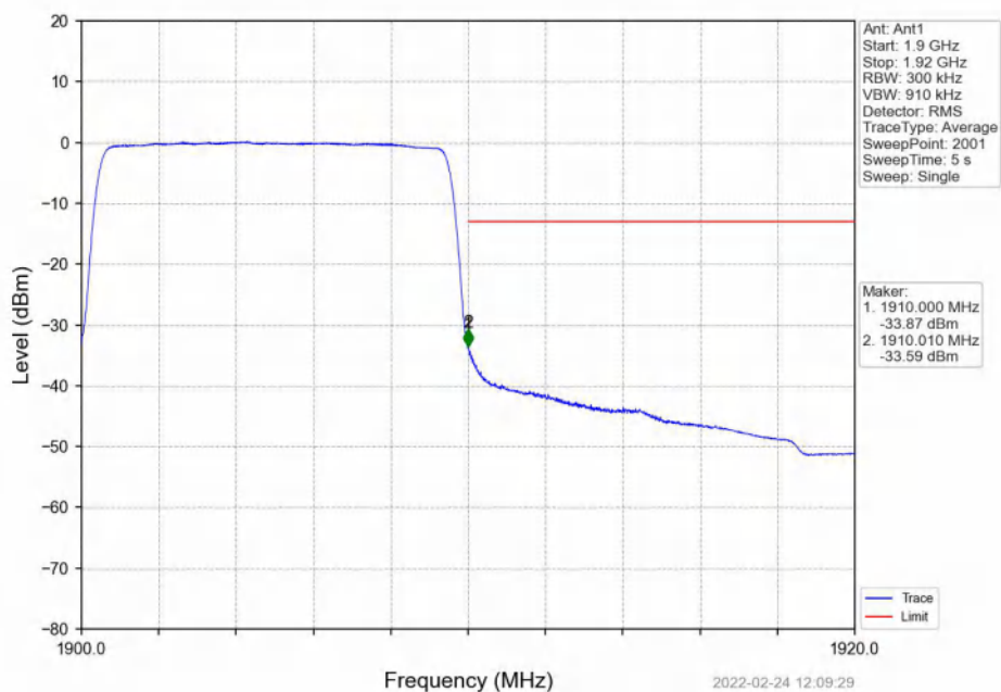
Band2_10MHz_QPSK_HCH_1905MHz_RB_50_0_NTNV
