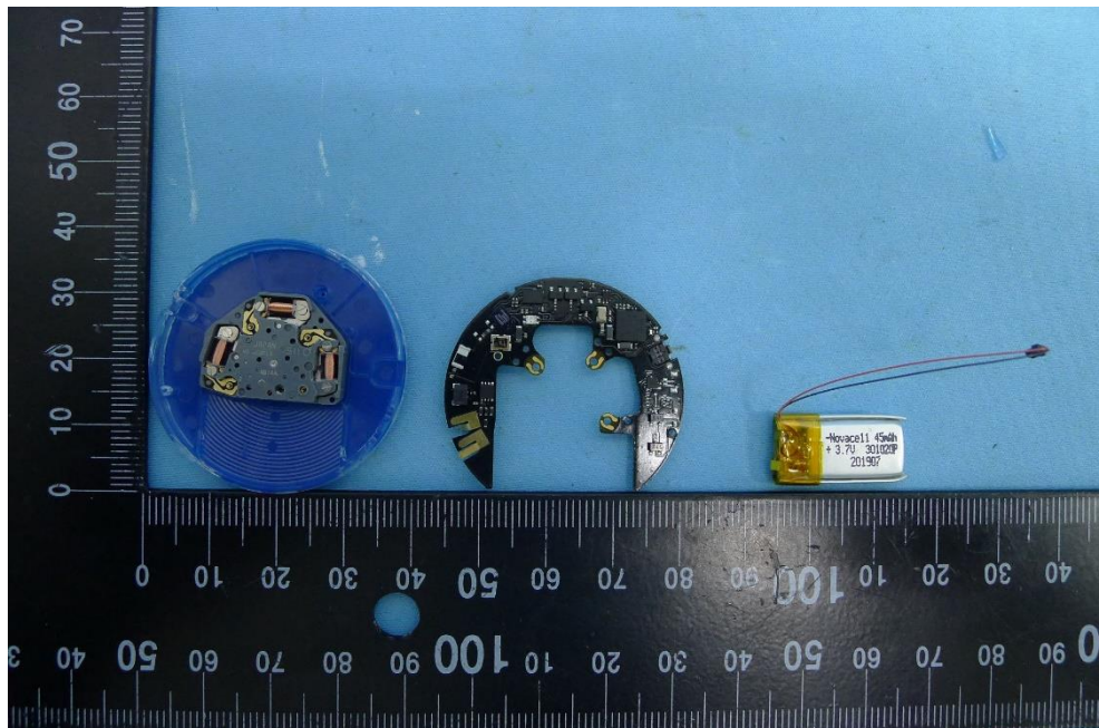
(6) EUT Photo
