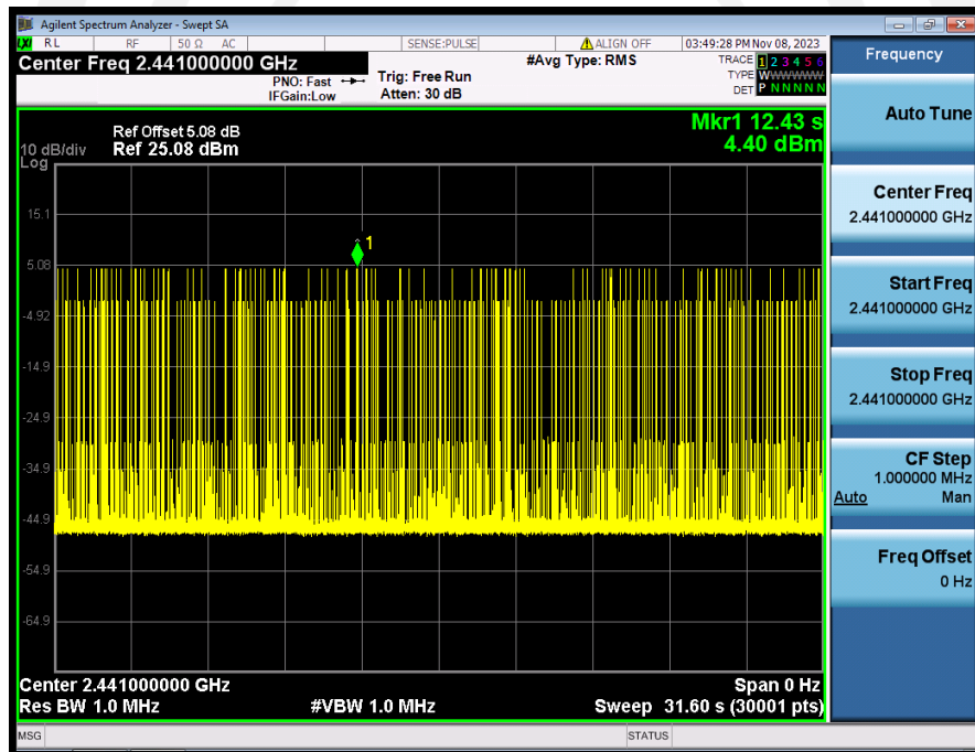
\pi/4 -DQPSK (2-DH5) 2441MHz
