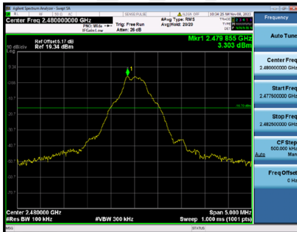
GFSK 2480MHz
