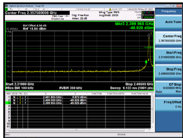
GFSK 2402MHz
