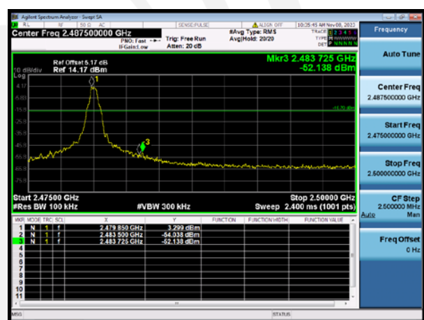
GFSK 2480MHz
