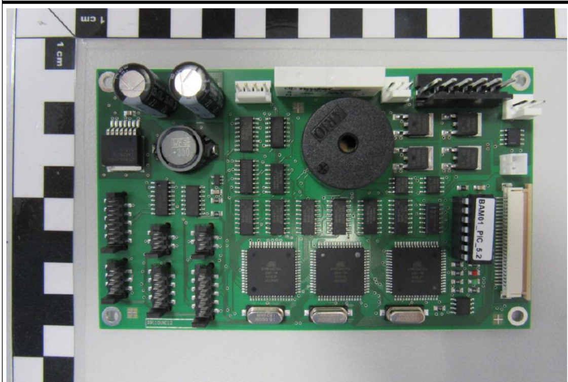
EUT PCB Top Side
