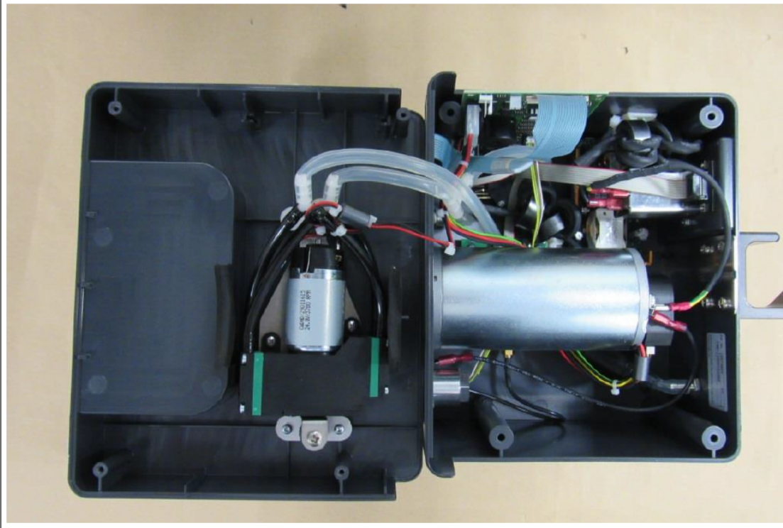
EUT Case Open
