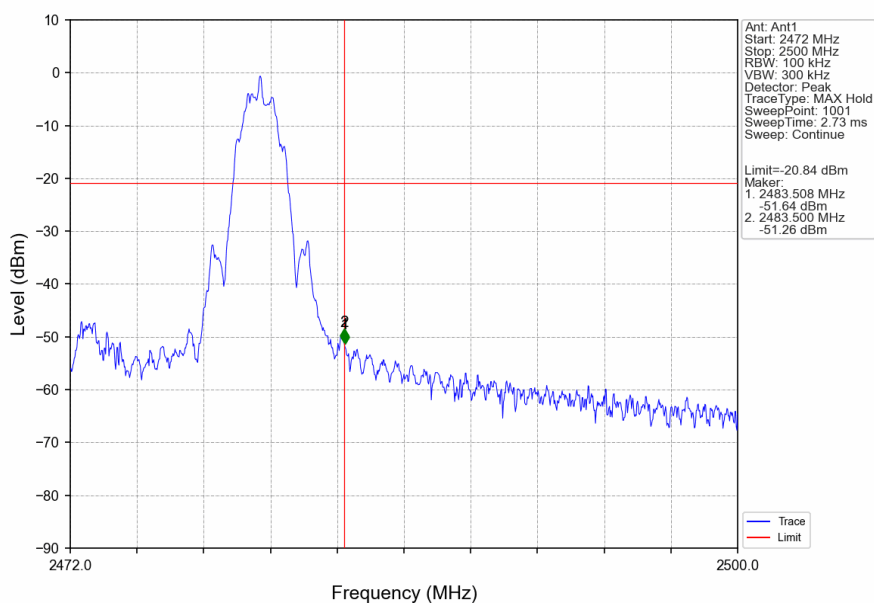
2M_HCH_2480MHz_Ant1_NTNV
