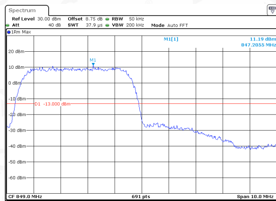
WCDMA 850-HCH
