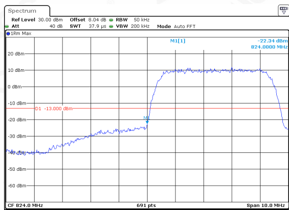
WCDMA 850-LCH
