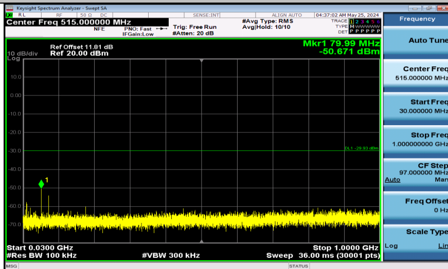
11G-Ant1-2462-30~1000-PASS
