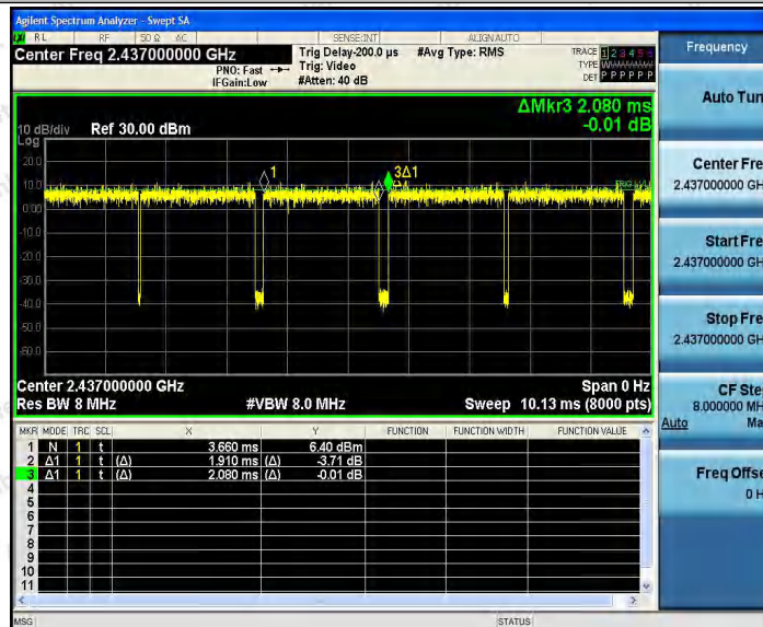
11N20_Ant2_2437
