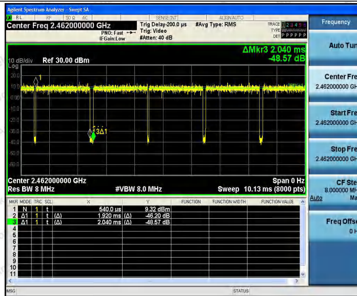
11N20_Ant3_2462
