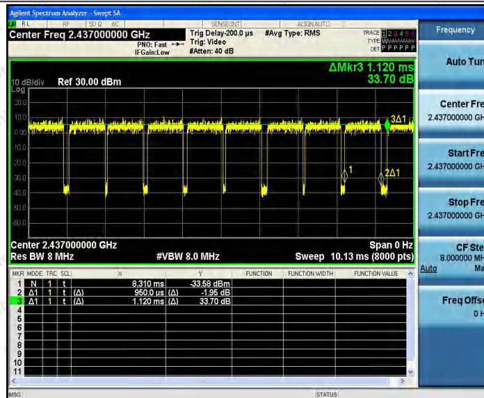
11N40_Ant3_2437
