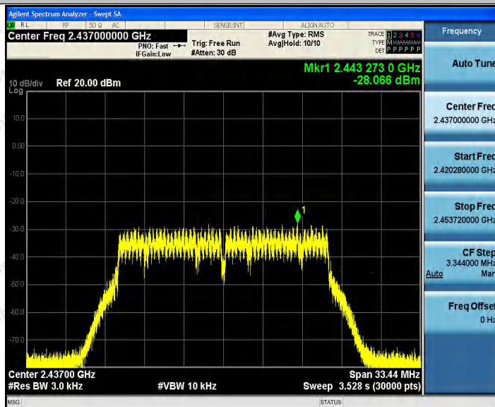
11N20_Ant2_2437
