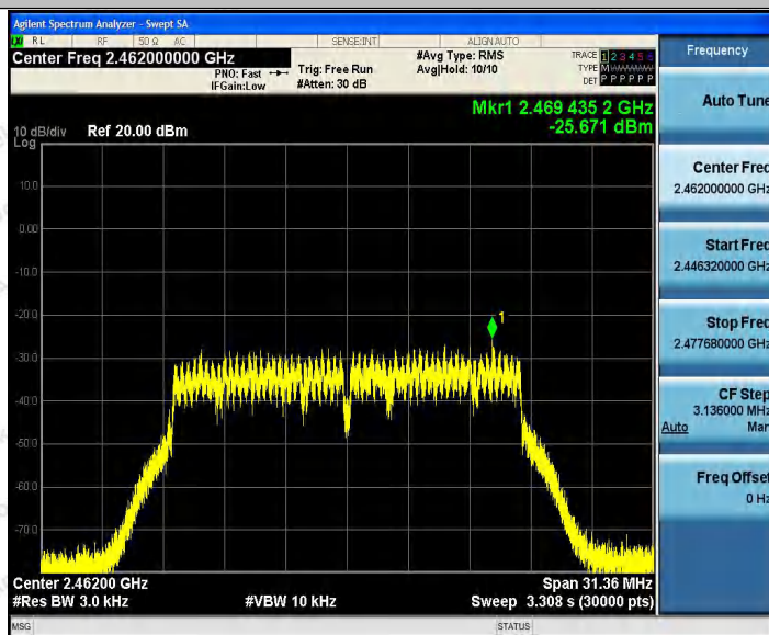
11N20_Ant3_2462
