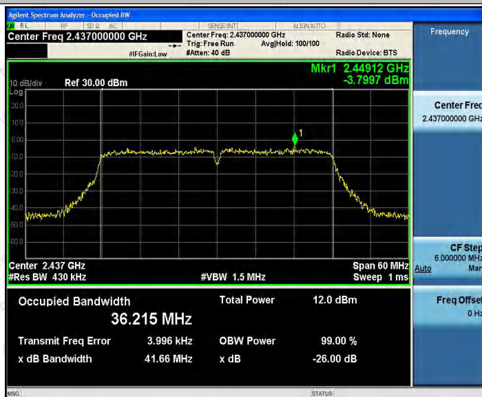
11N40_Ant3_2437
