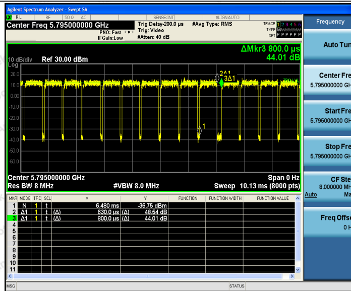
11N40SISO_Ant2_5795
