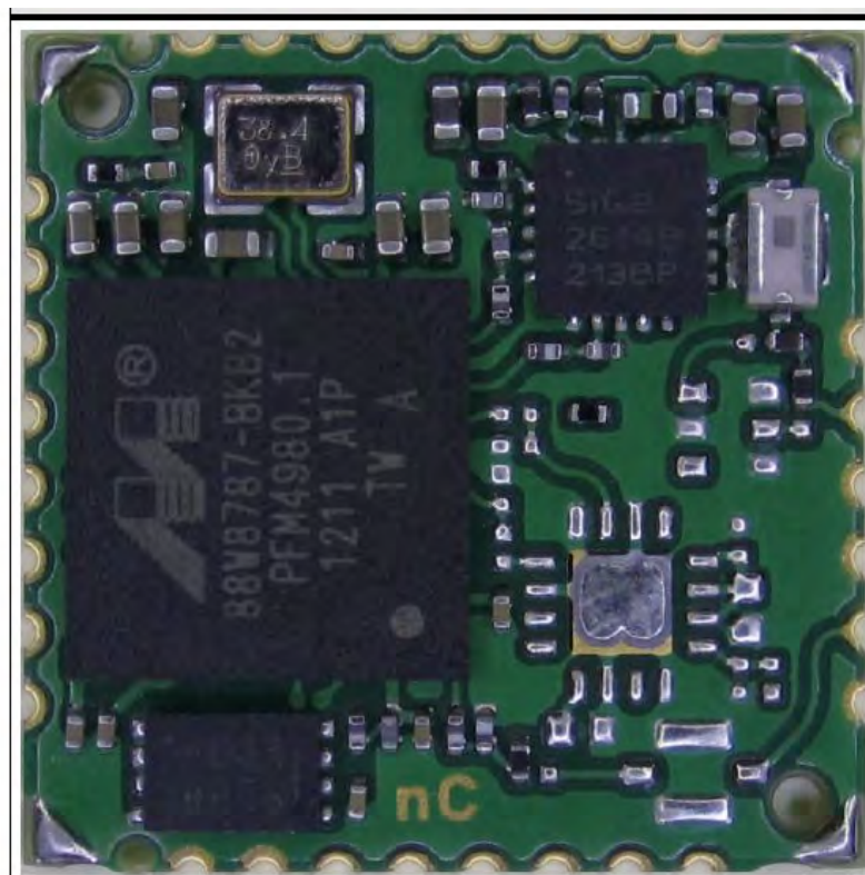
W-LAN Module w-o- label:
