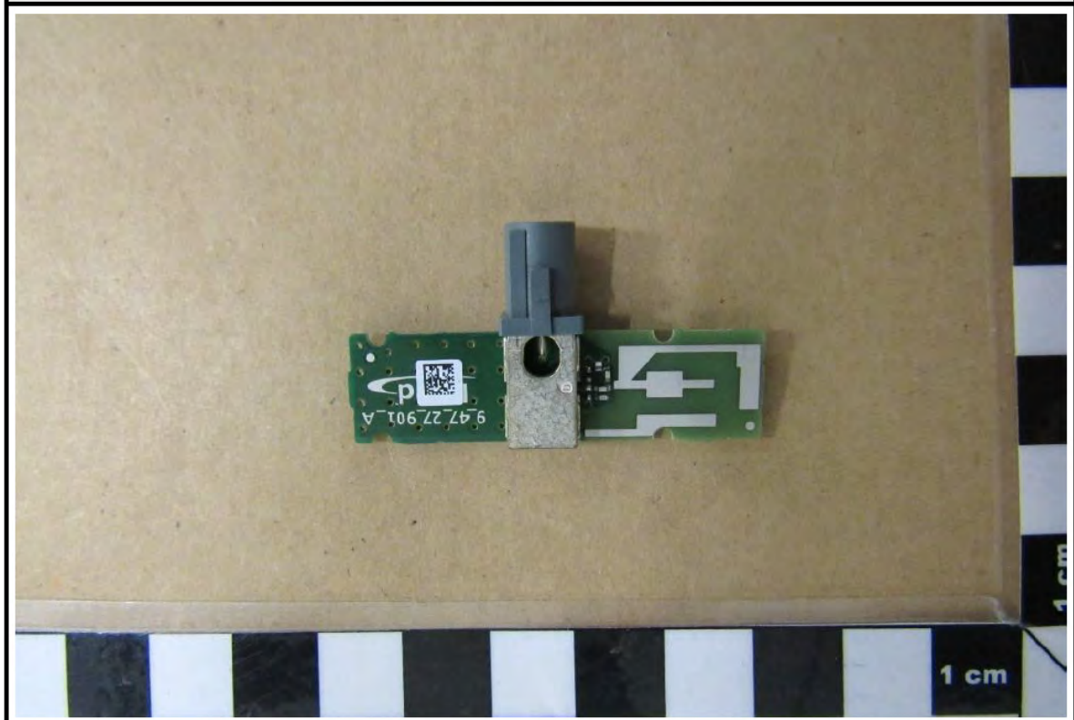
AE: WiFi antenna PCB top
