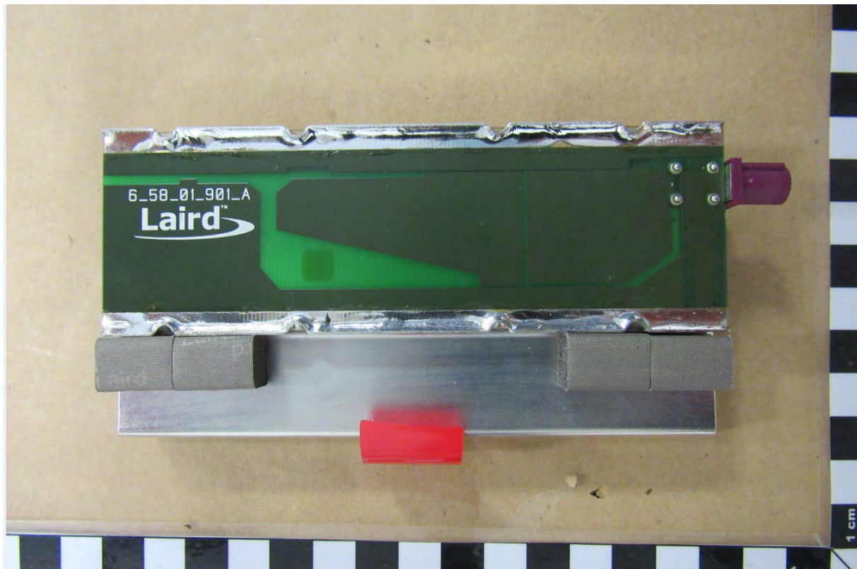
AE: LTE Antenna back
