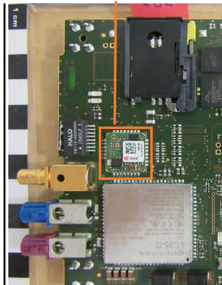
W-LAN Module w-o- label:
