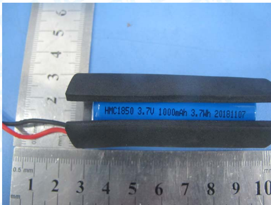
Photo 14 Battery Parameter
