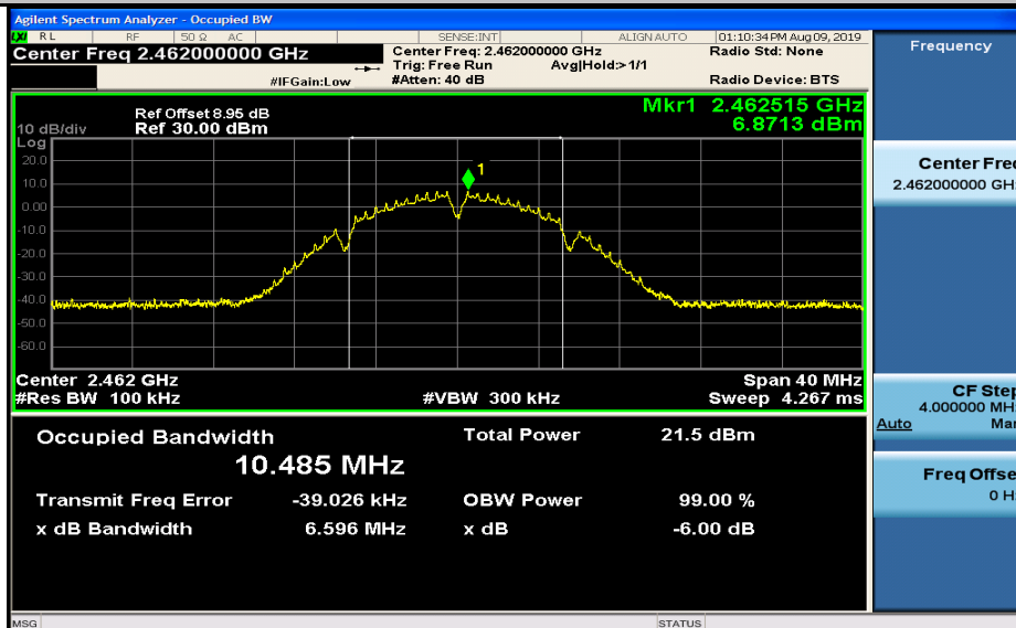
6dB Bandwidth_11B_2462_Ant2
