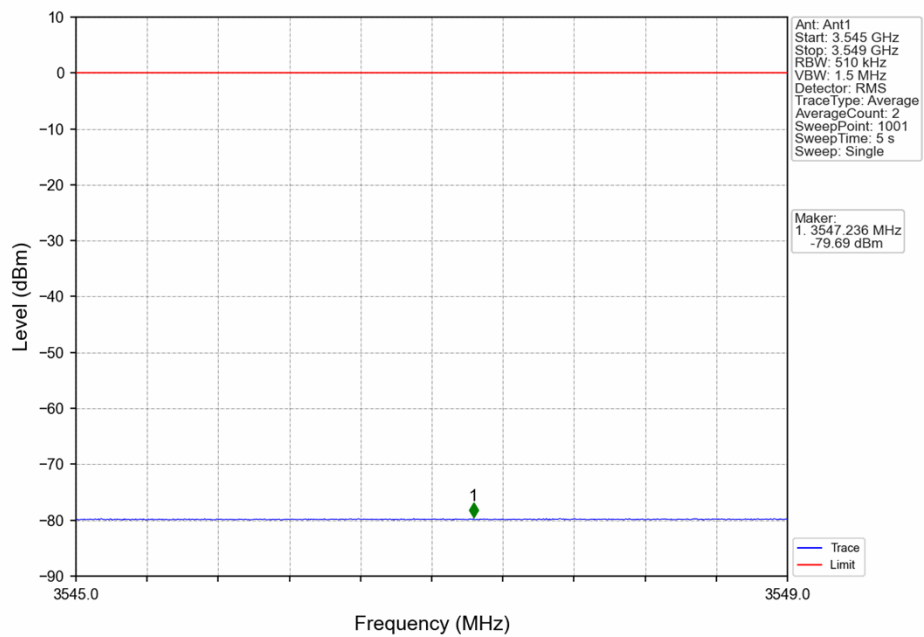
n48_30kHz_SISO_NTNV_10MHz_CP-OFDM_QPSK_3555MHz_Edge_1RB_Left
