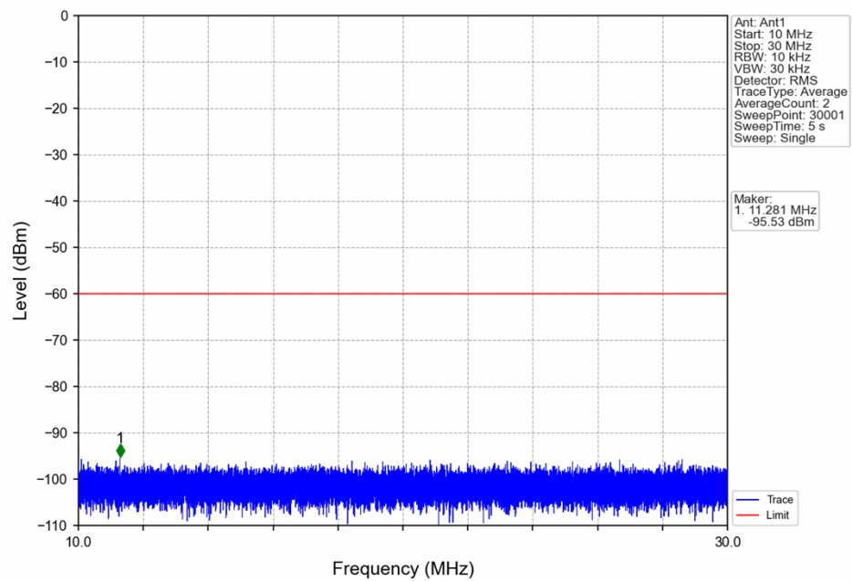
n48_30kHz_SISO_NTNV_10MHz_CP-OFDM_QPSK_3555MHz_Edge_1RB_Left
