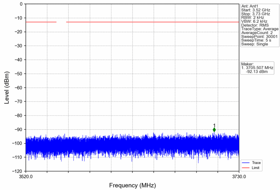
n48_30kHz_SISO_NTNV_10MHz_CP-OFDM_QPSK_3555MHz_Inner_1RB_Left
