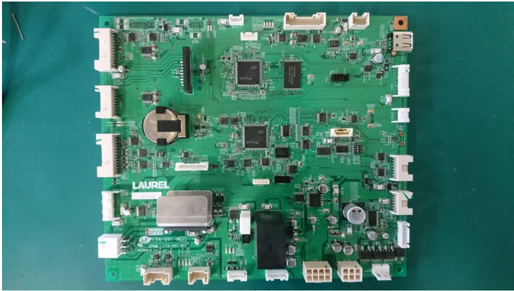
1TA-001-B(Component Side)
