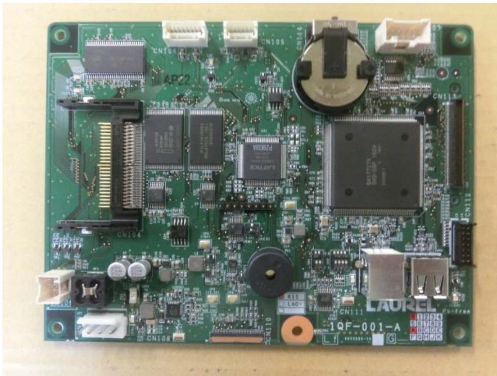
1QF-001-A (Component Side)
