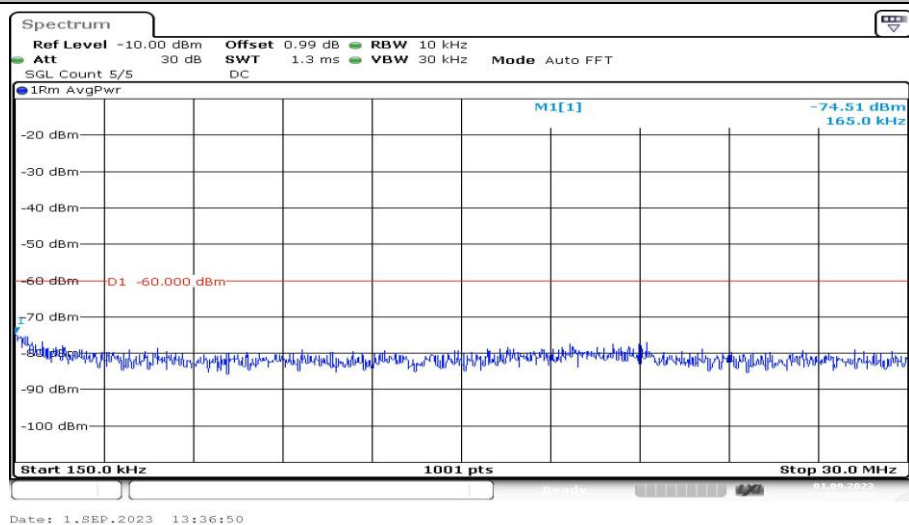
Band40-10MHz-QPSK-38750-1RB#0-Range2:0.15~30MHz-PASS
