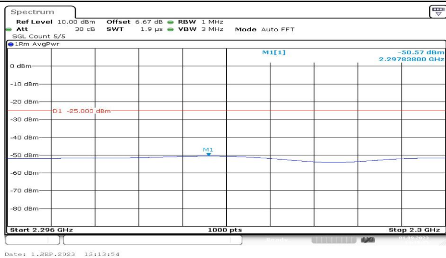
Band40-5MHz-QPSK-38775-1RB#0-Range7:2296~2300MHz-PASS
