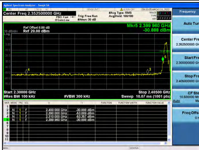
BLE_2M_Ant1_Low_2402
